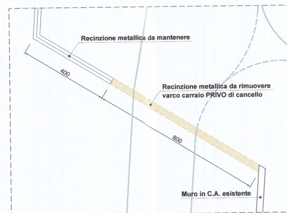
PARTICOLARE A - PIANTE NUOVO VARCO CARRAIO Scala 1:100
