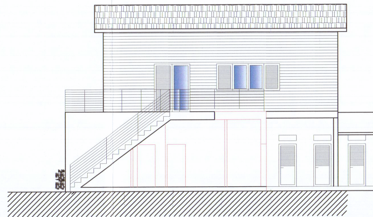
SEZIONE C-C
