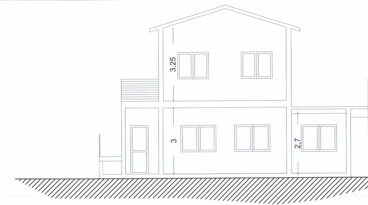
SEZIONE B-B
