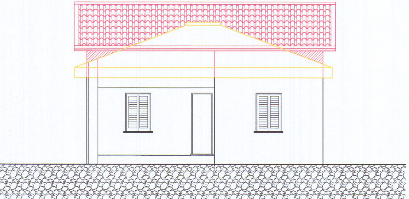
PROSPETTO LATO MONTI
