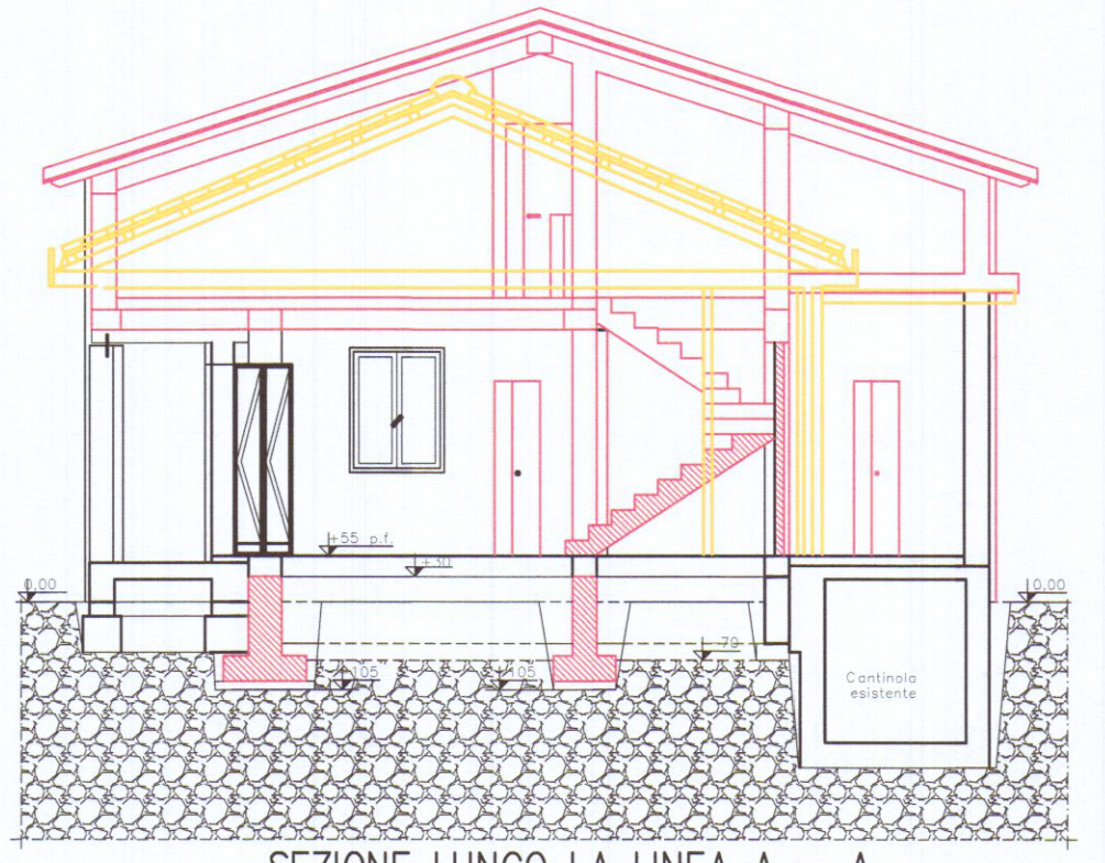
SEZIONE LUNGO LA LINEA A - A
