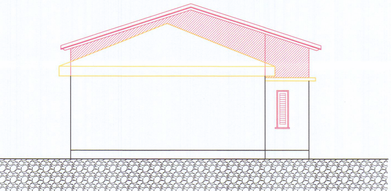
PROSPETTO LATO SARZANA
