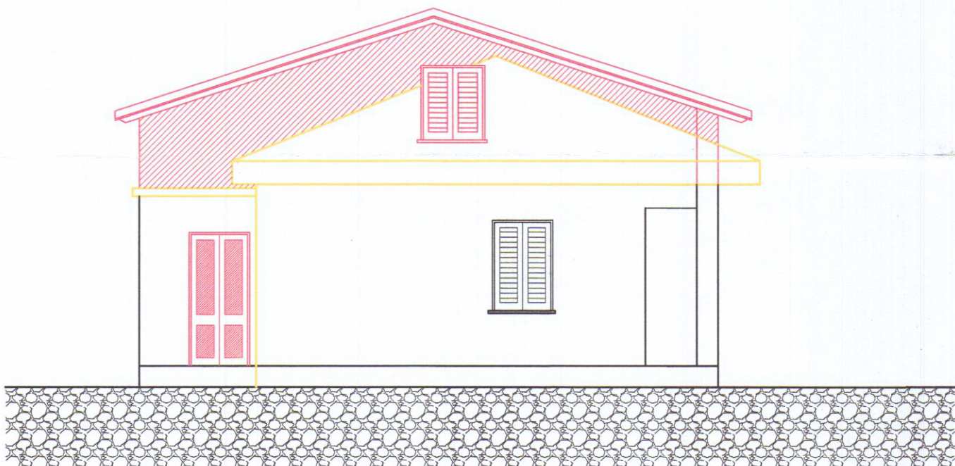
PROSPETTO LATO VIEREGGIO
