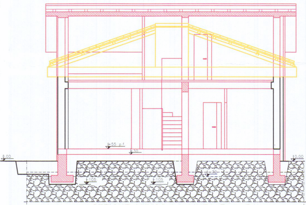
SEZIONE LUNGO LA LINEA B - B
