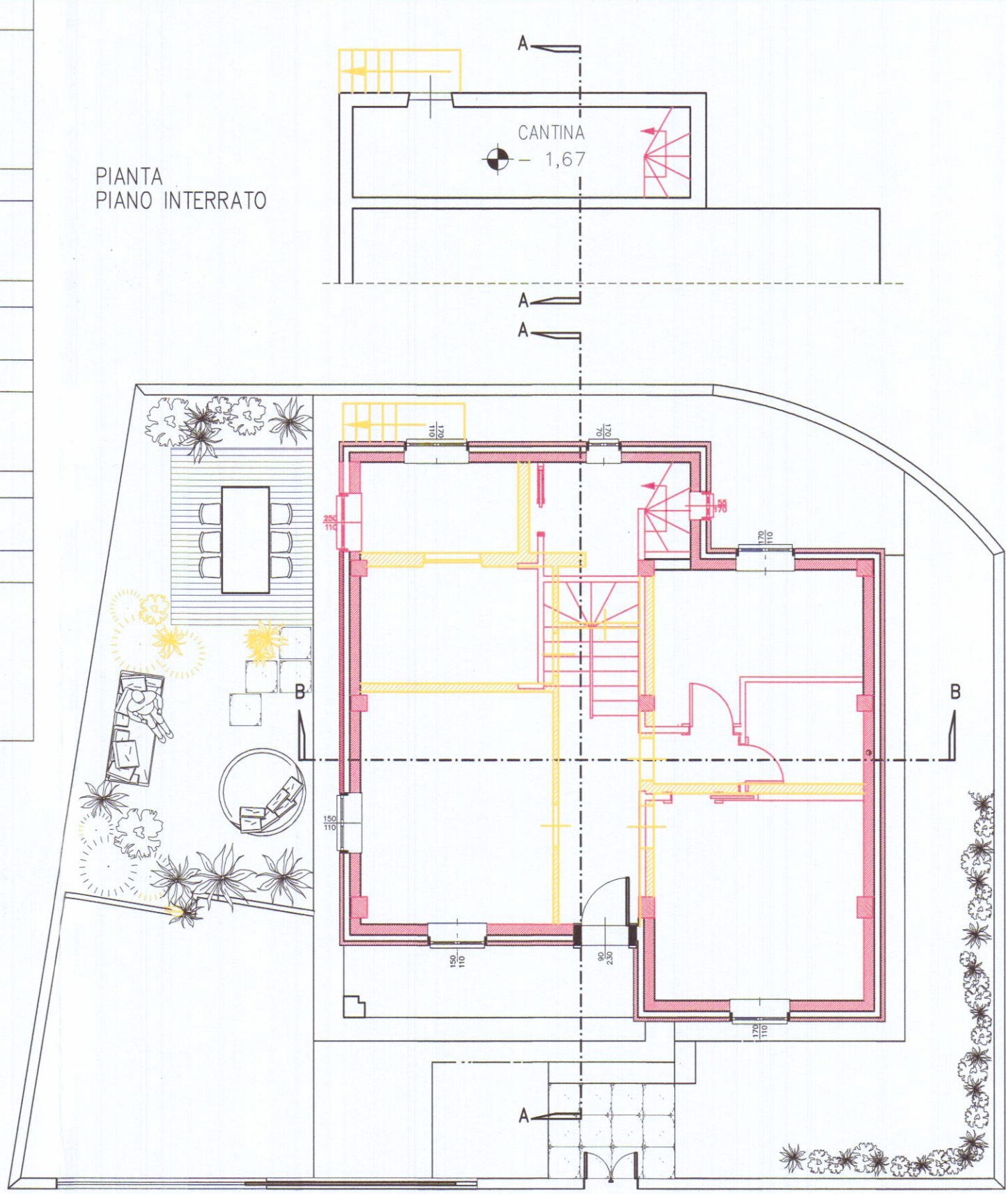
PIANTA PIANO TERRA VIA PROVINCIALE AVENZA SARZANA
