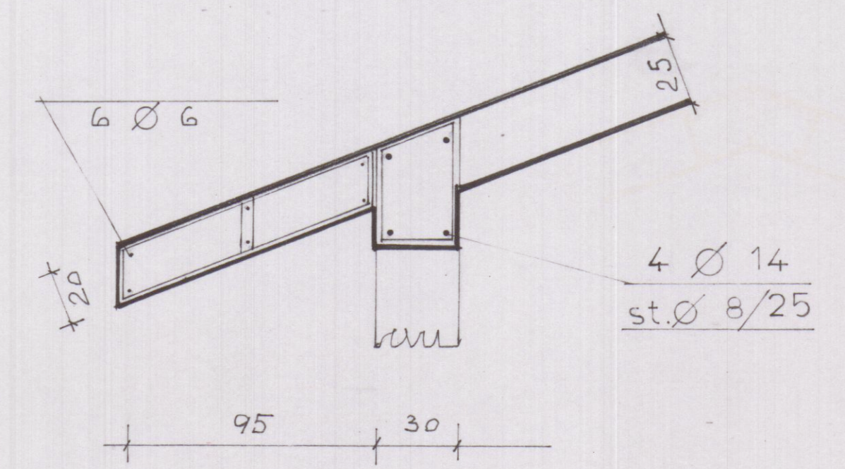
SCALA = 1:20 - PARTICOLARE DI GRONDA -
