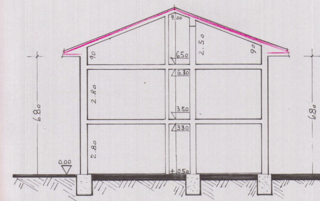
SEZIONE X-X
