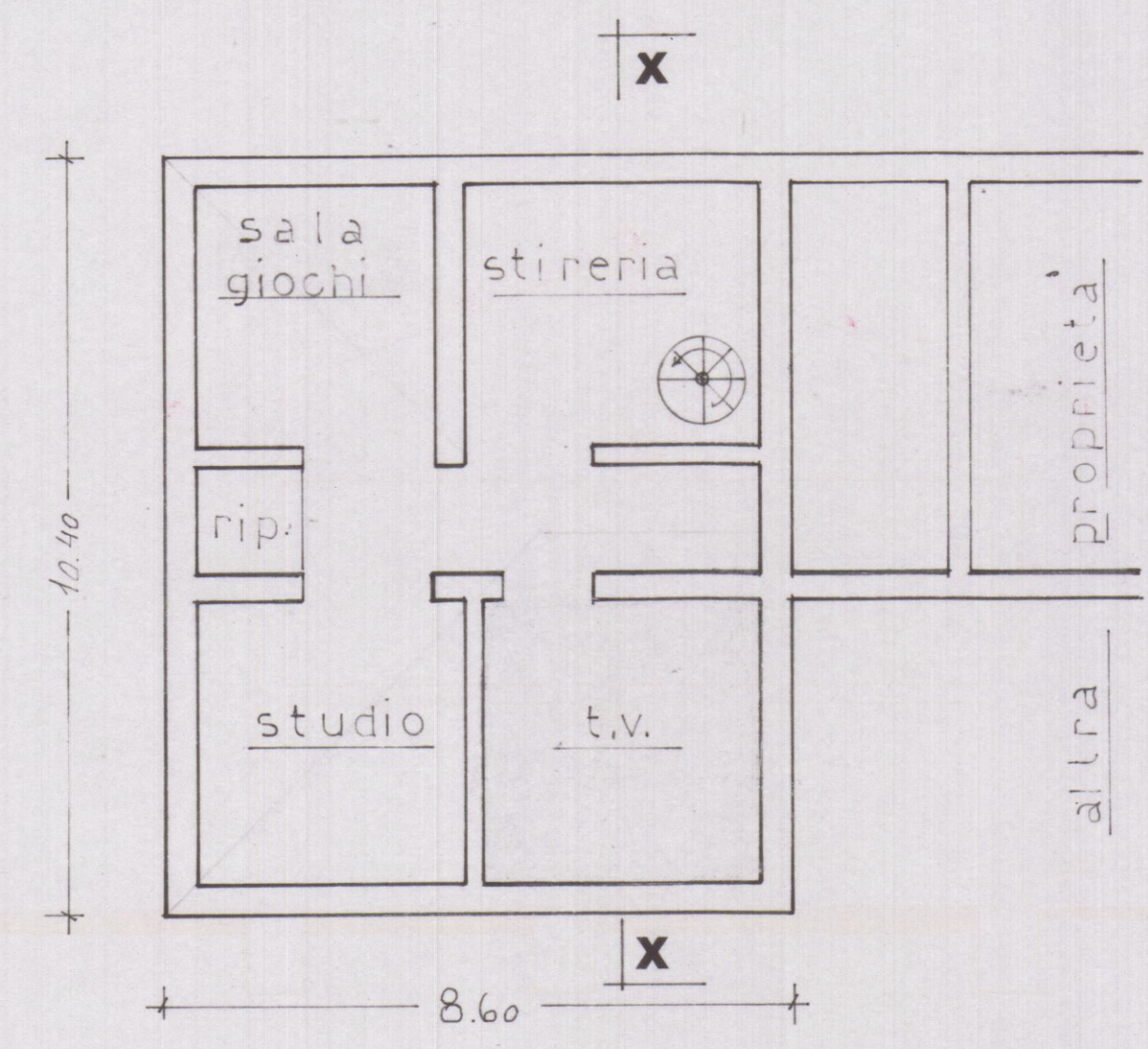
PIANTA SOTTOTETTO
