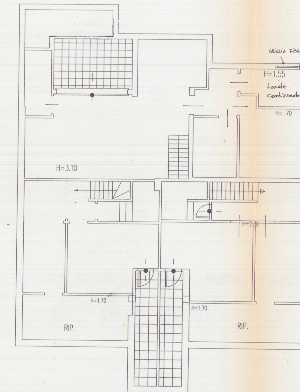
PIANO ATTICO Sotto Hotel
