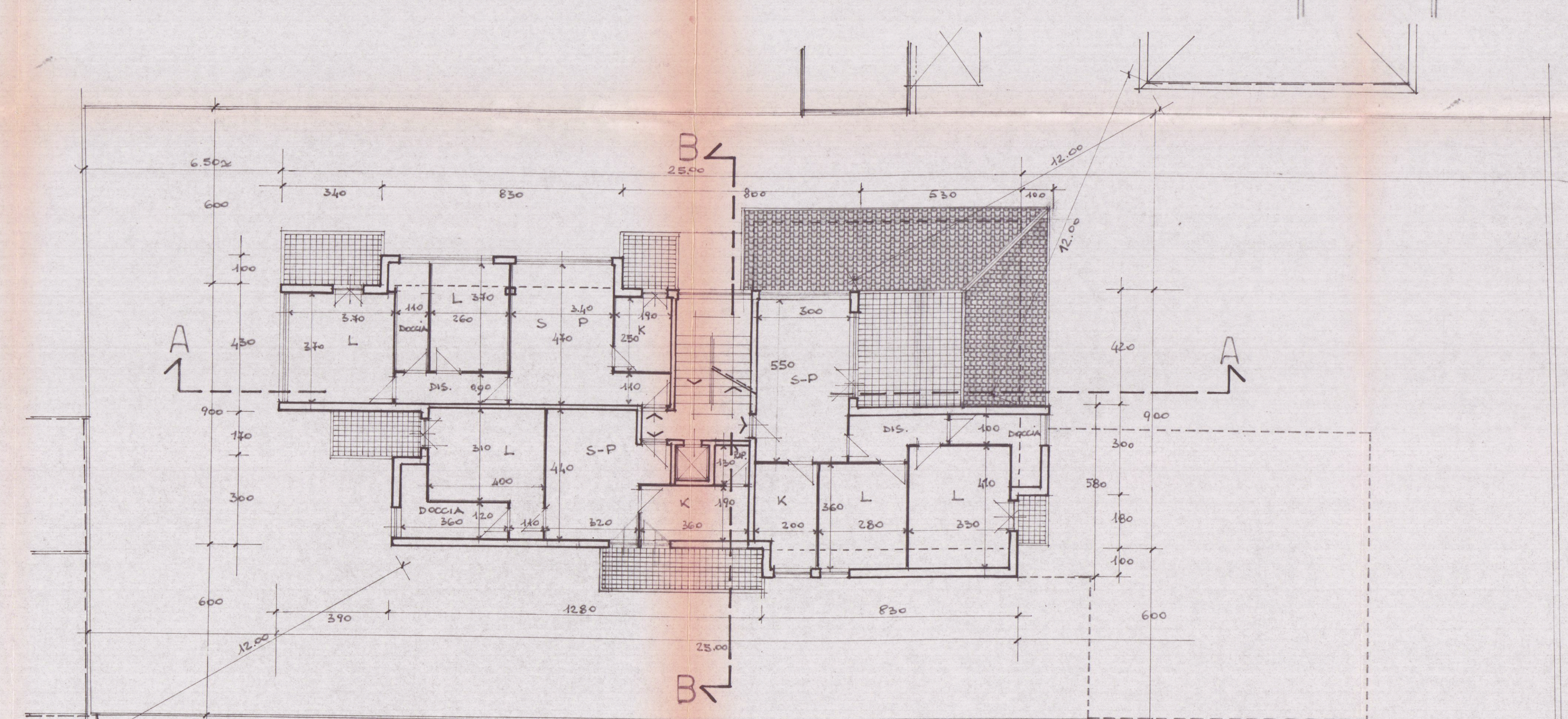
PIANO 2° RAPP. 1:100
