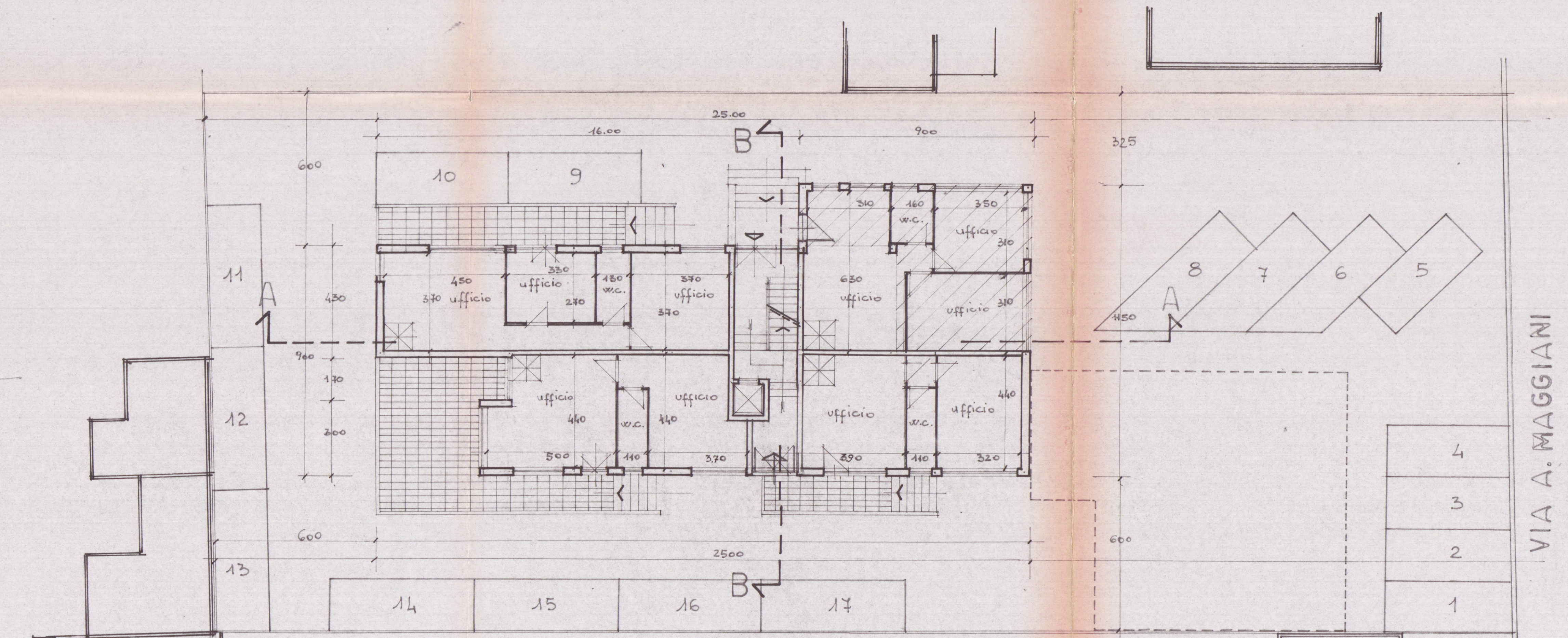
PIANO RIALZATO RAPP. 1:100
