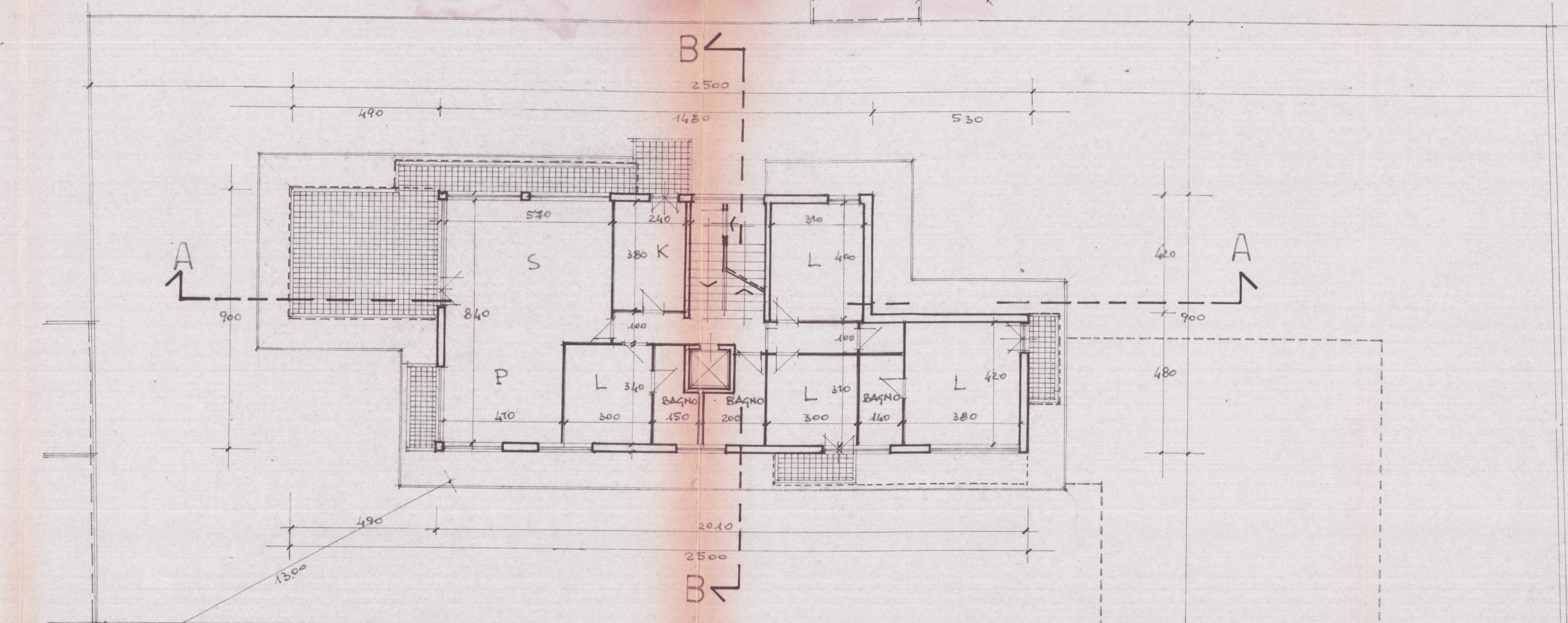
PIANO 4° RAPP. 1:100
