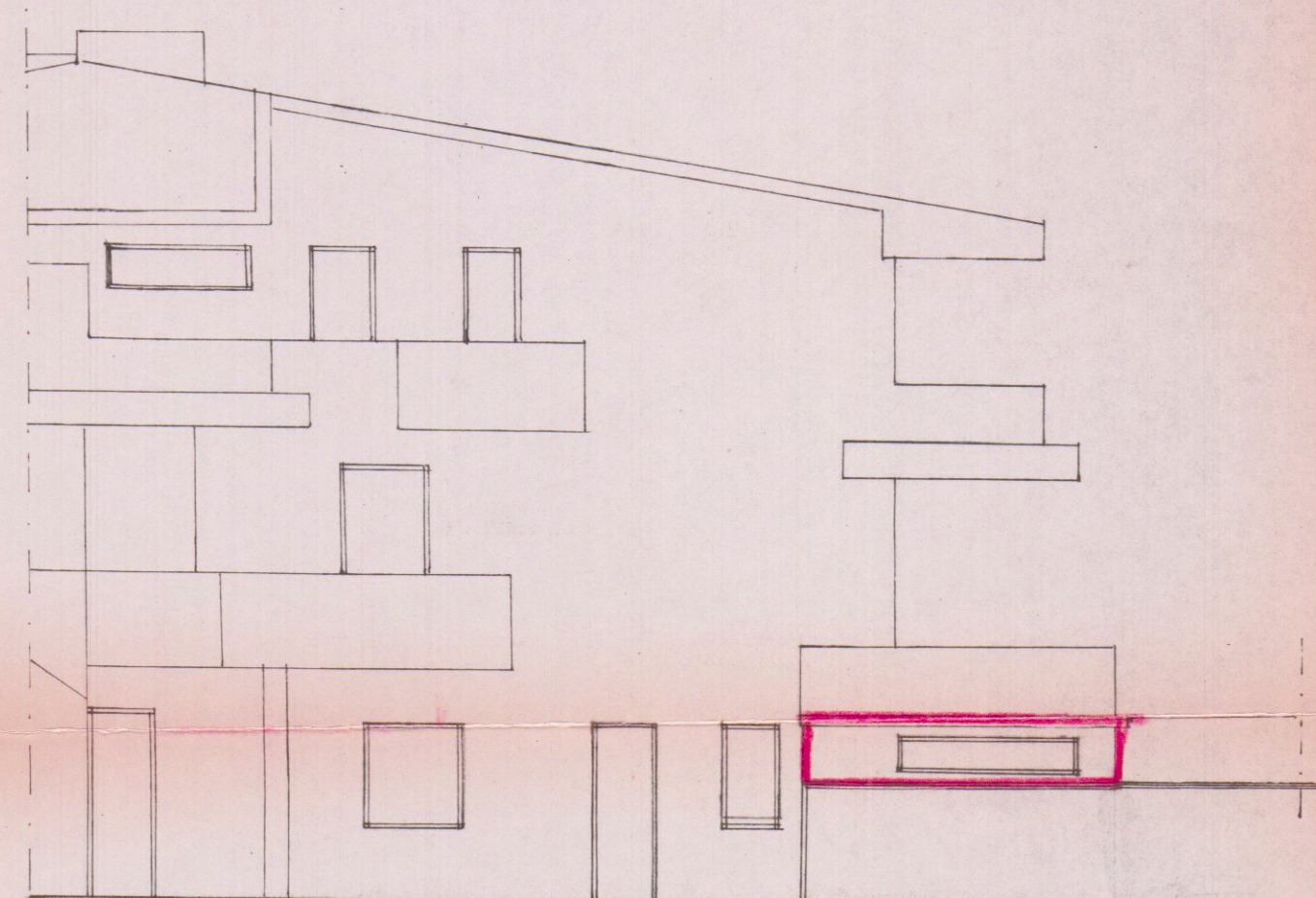
PROSPETTO NORD-OVEST
