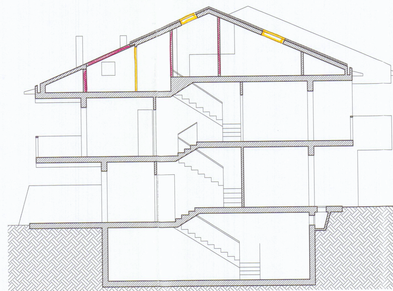
SEZIONE
