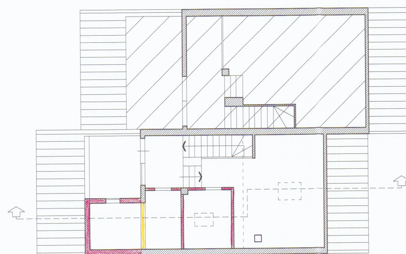
PIANO SOTTOTETTO
