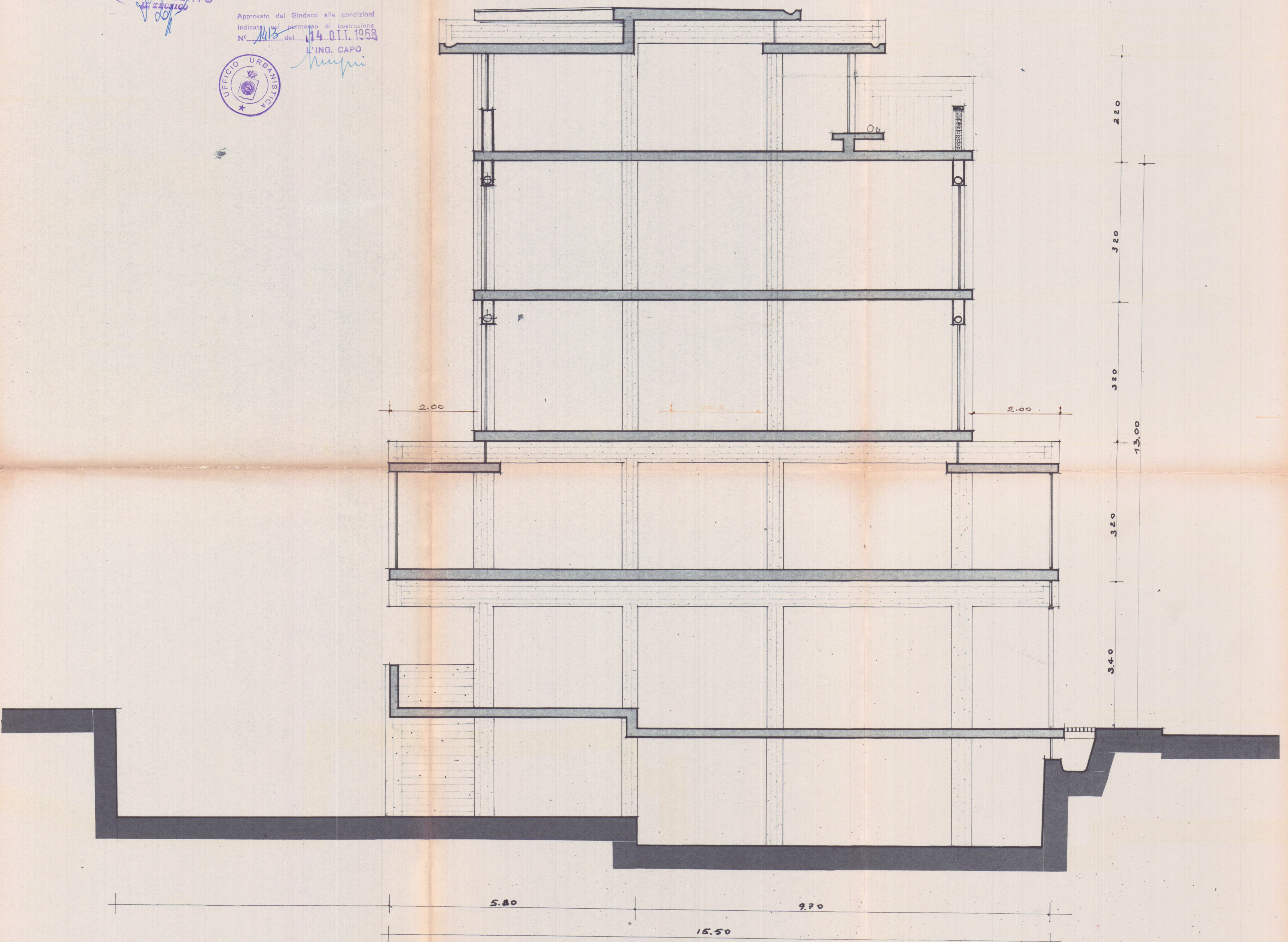
SEZIONE C - D
