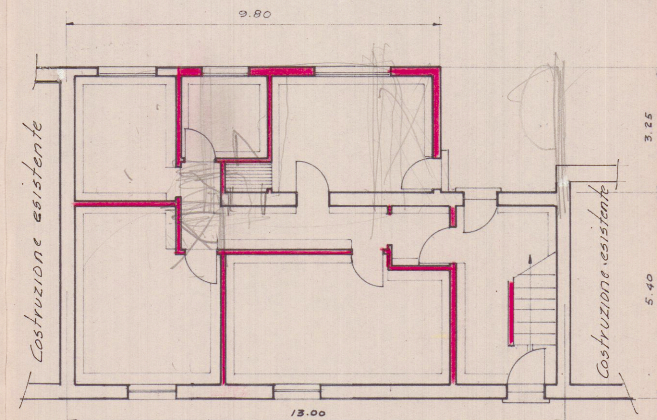
NUOVO PROGETTO PIANO TERRA
