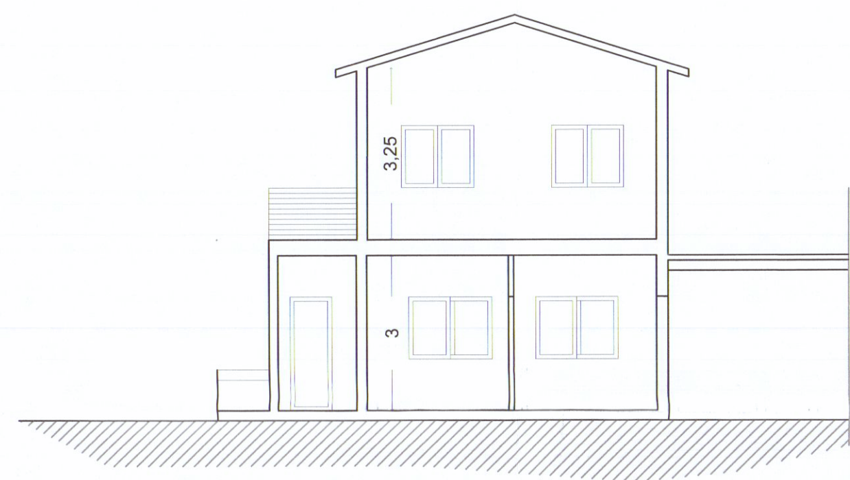
SEZIONE B-B
