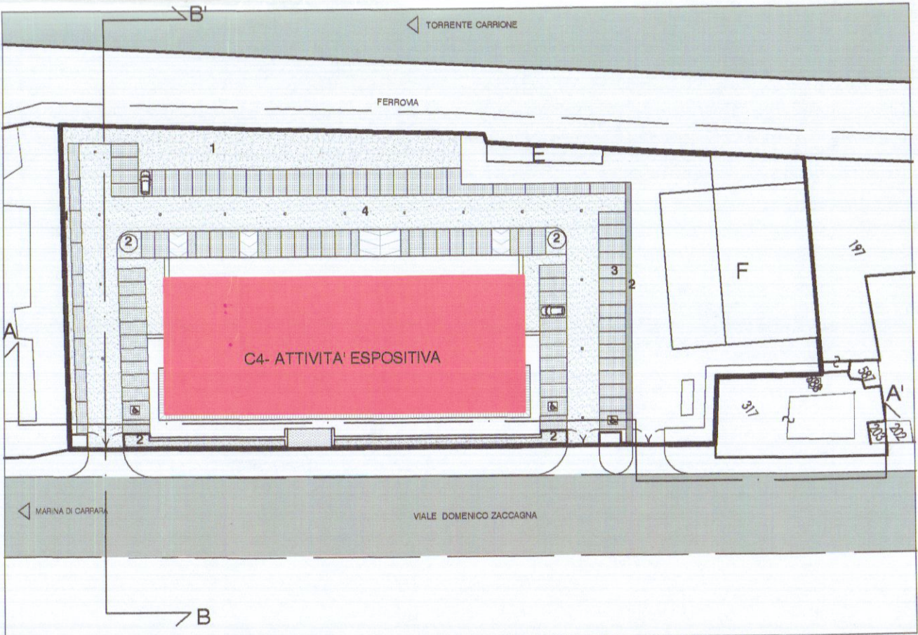
Planimetria di progetto 1:1000 rosso: nuova costruzione
