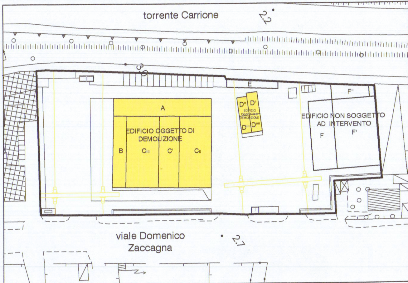
Planimetria dello stato di fatto 1:1000 giallo : demolizioni
