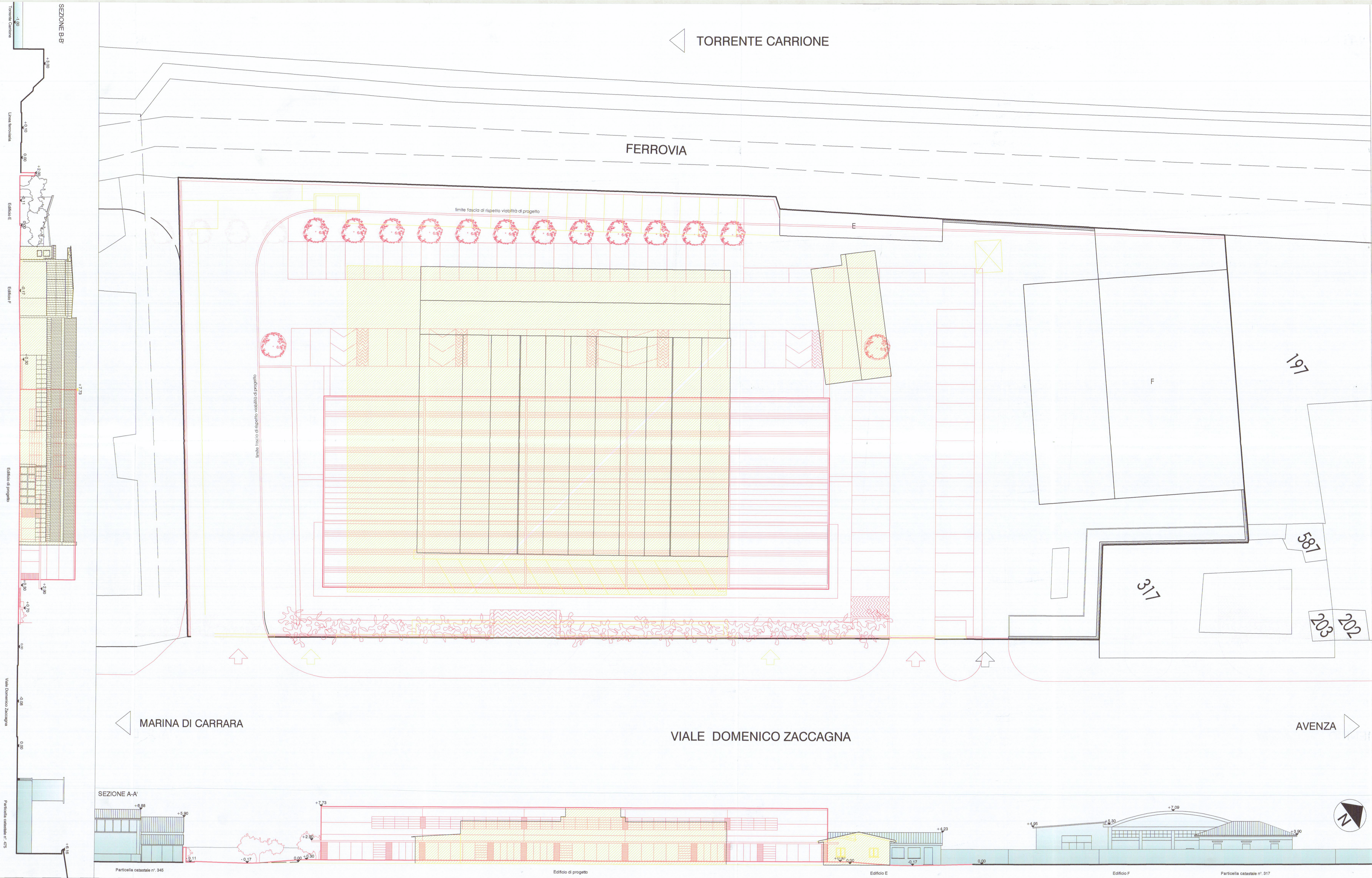
Planimetria di progetto 1:1000 rosso: nuova costruzione
