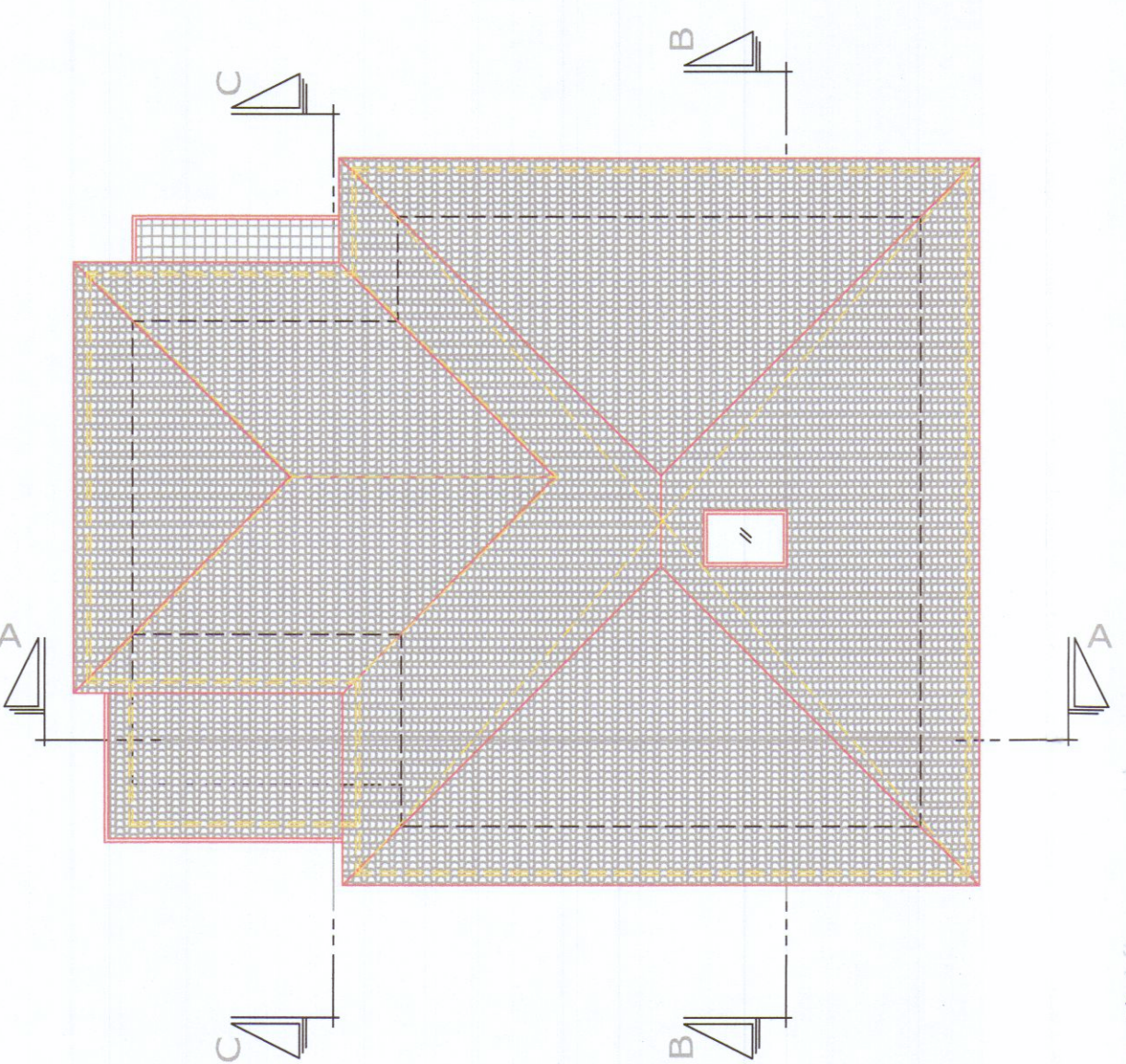
PIANO COPERTURA
