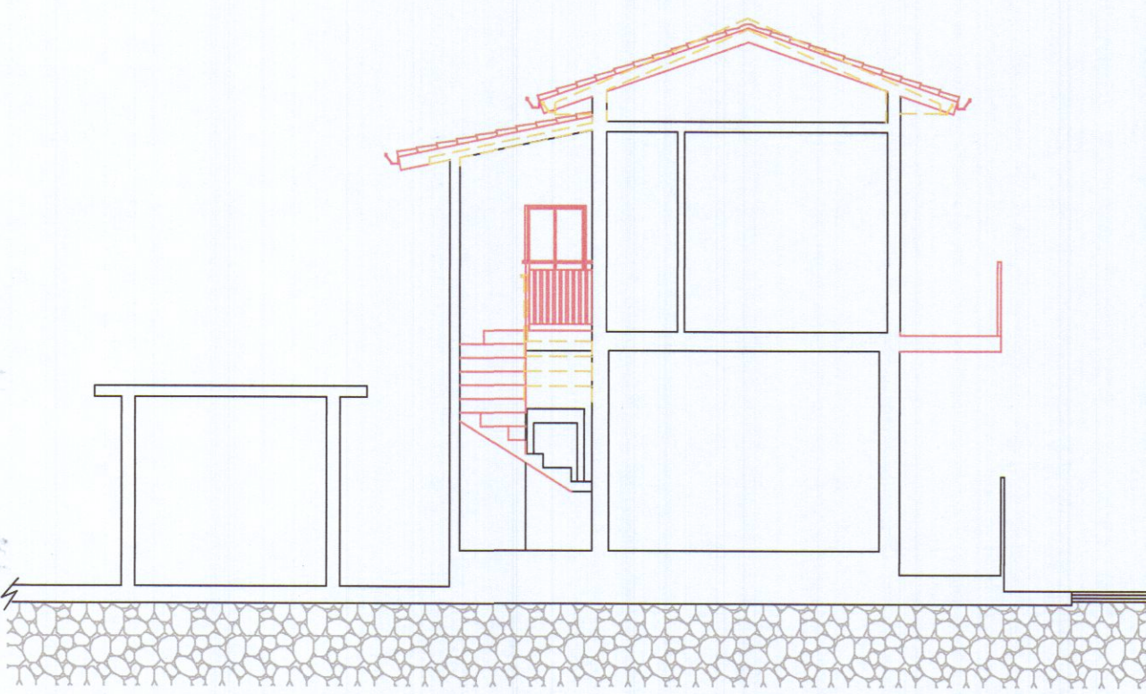
SEZIONE C-C
