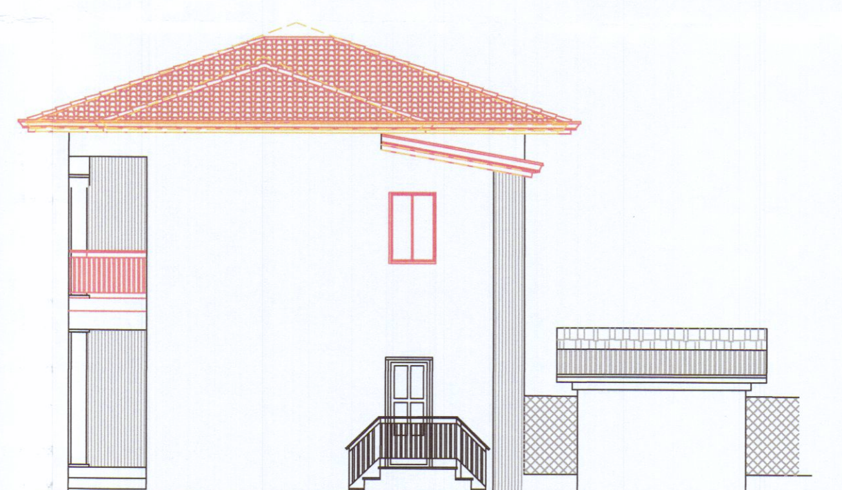
PROSPETTO EST
