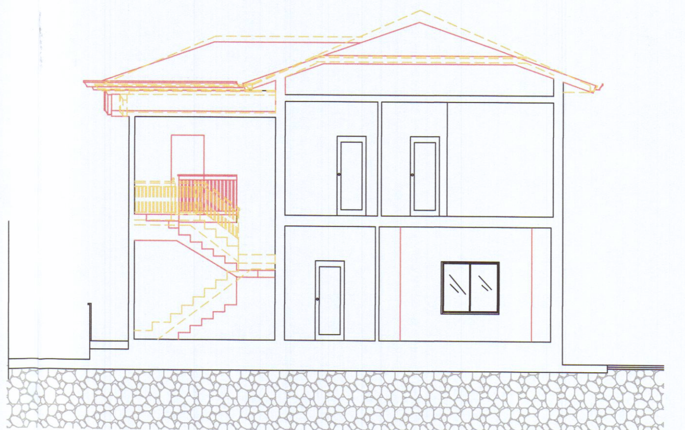
SEZIONE A-A
