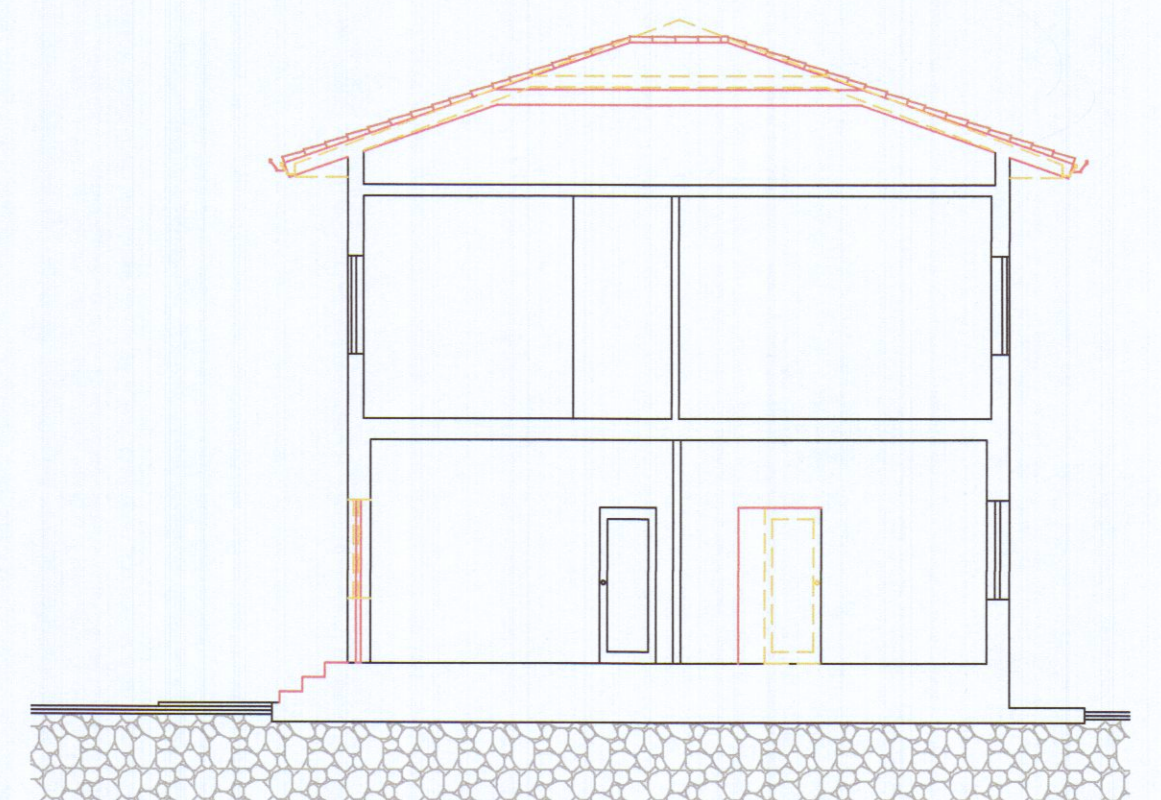
SEZIONE B-B
