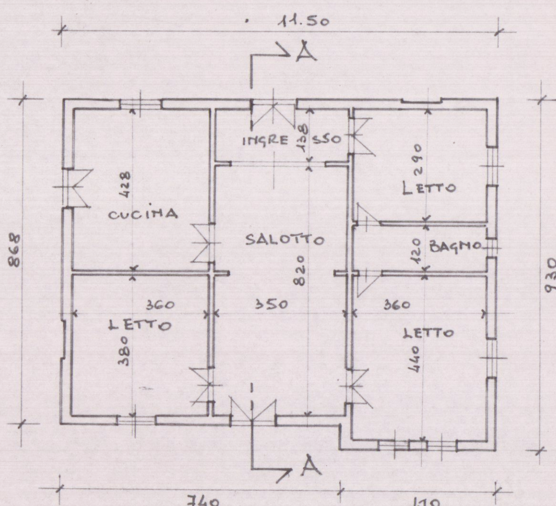
PIANTA PIANO TERRA RAPP. 1:100
