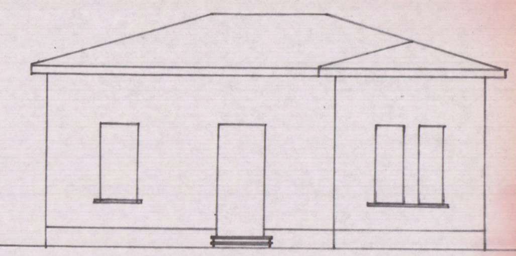
FRONTE SUD RAPP. 1:100
