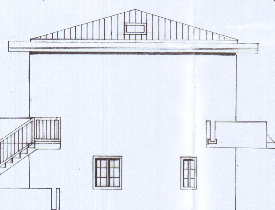
PROSPETTO SUD DA PROGETTO
