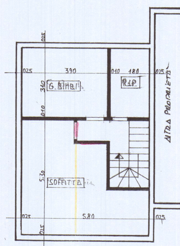
PIANTA SOTTOTETTO DA PROGETTO
