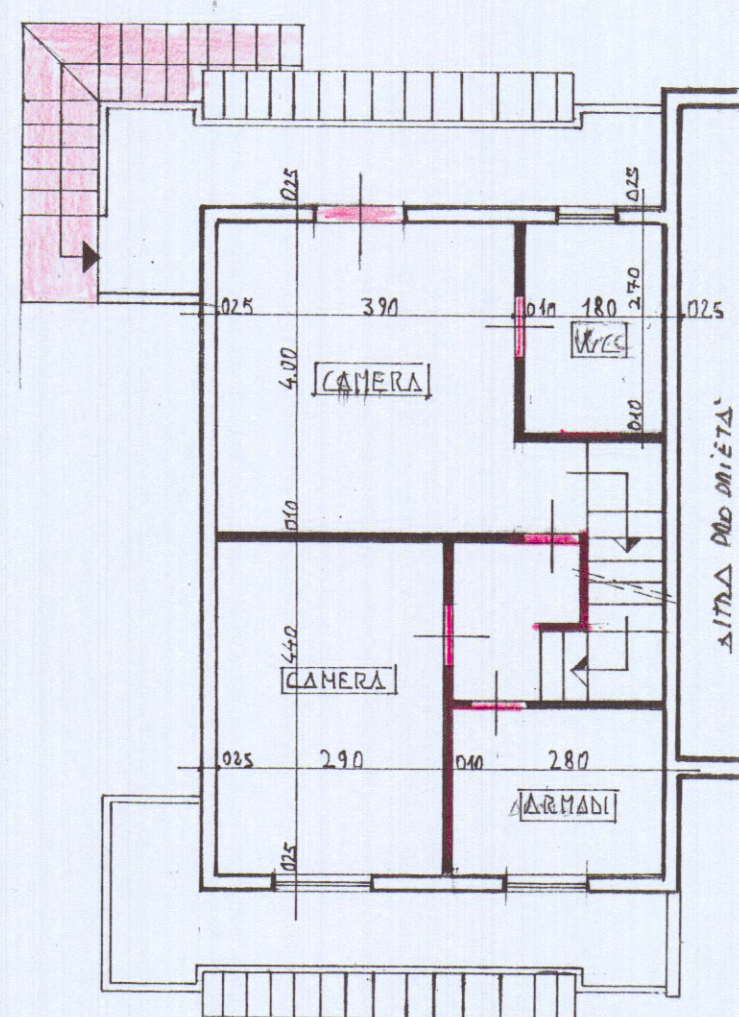
PIANTA P. PRIMO DA PROGETTO
