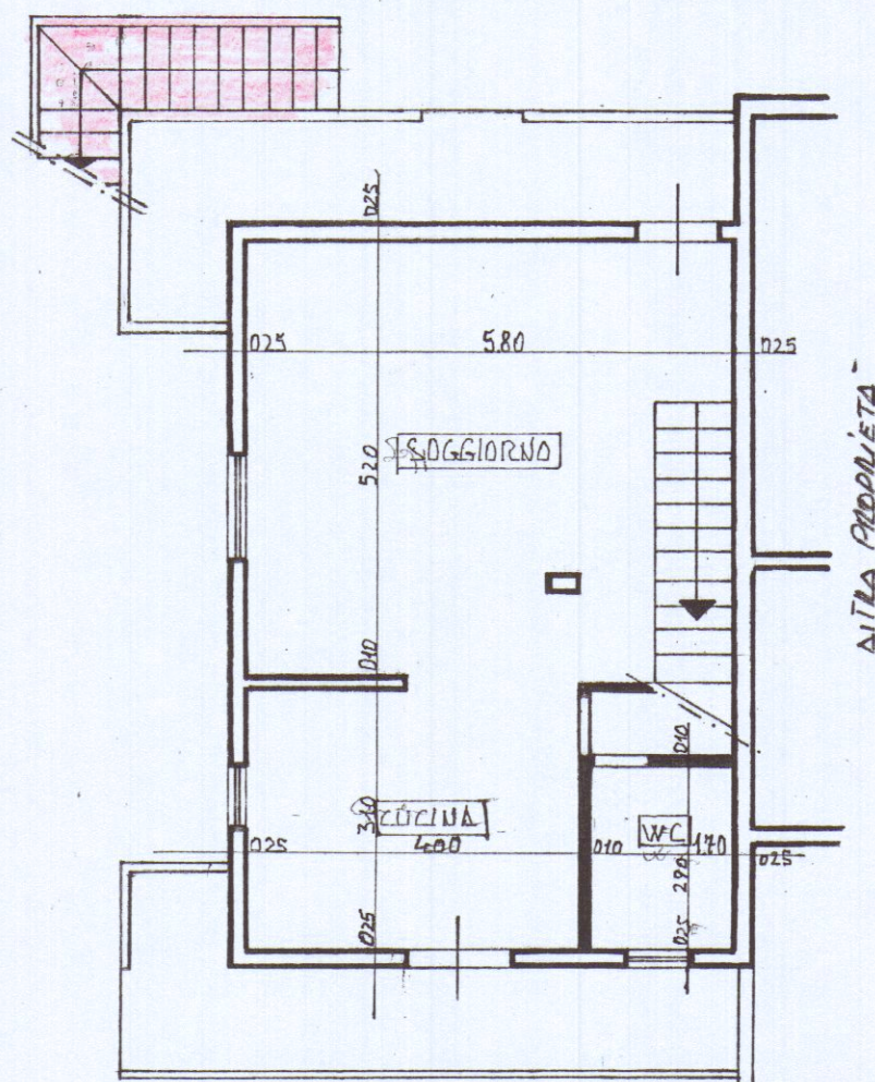
PIANTA P. TERRA DA PROGETTO
