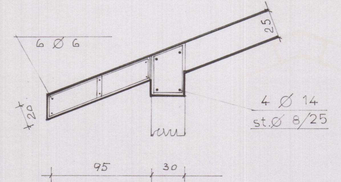
SCALA = 1:20 - PARTICOLARE DI GRONDA -
