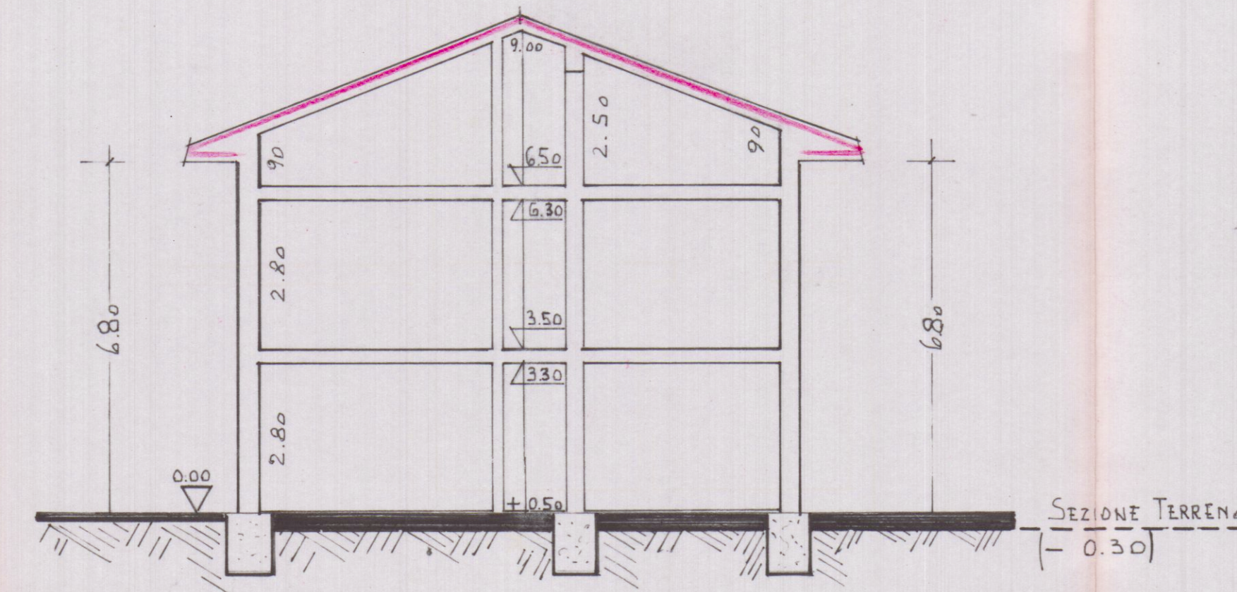
SEZIONE X-X
