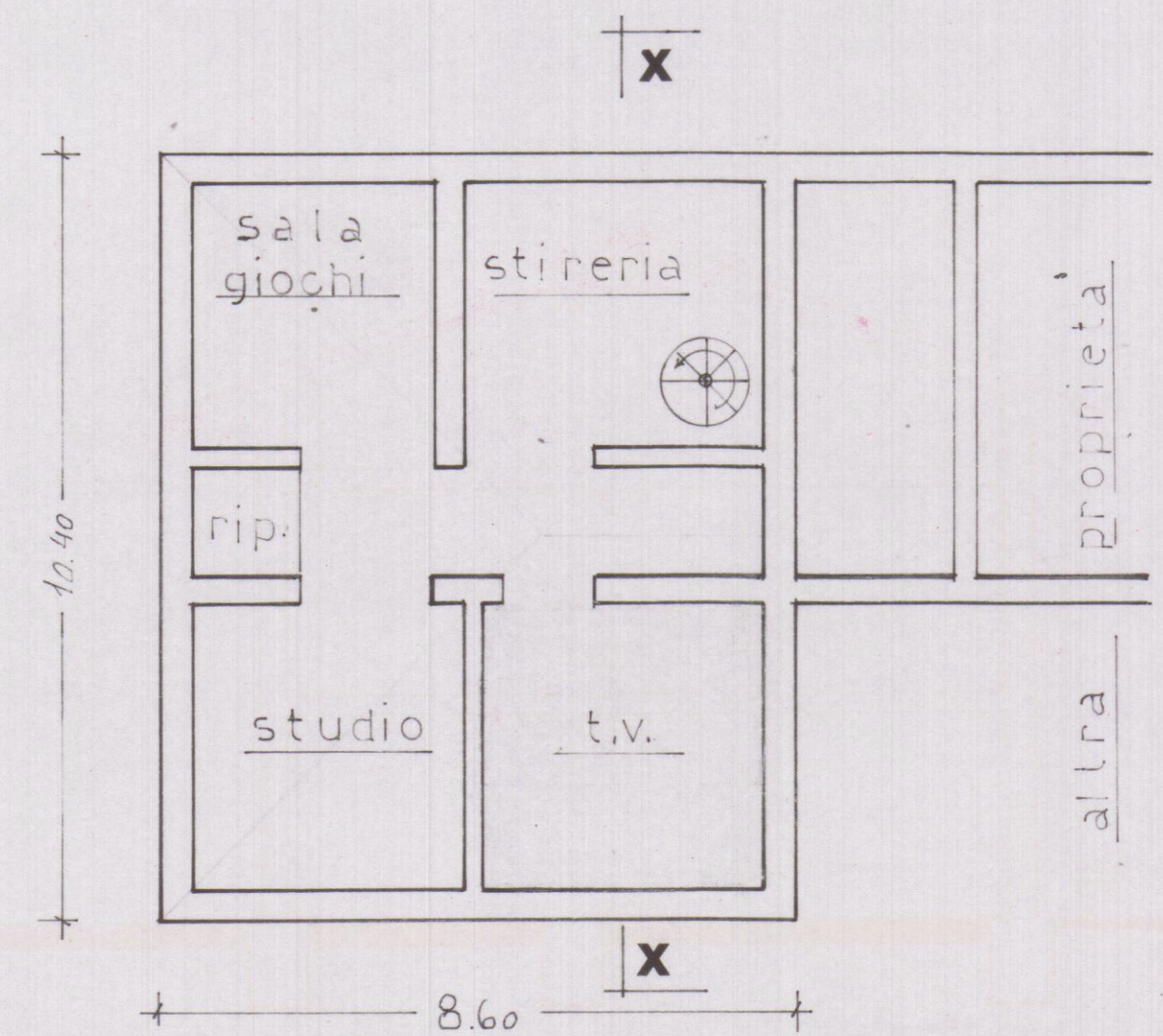
PIANTA SOTTOTETTO
