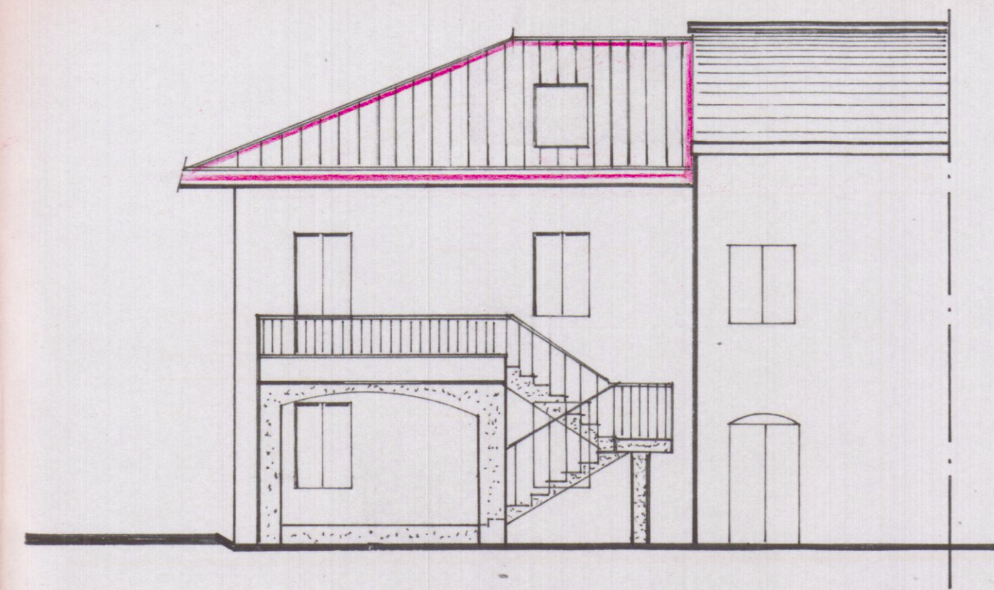
-PROSPETTO-
