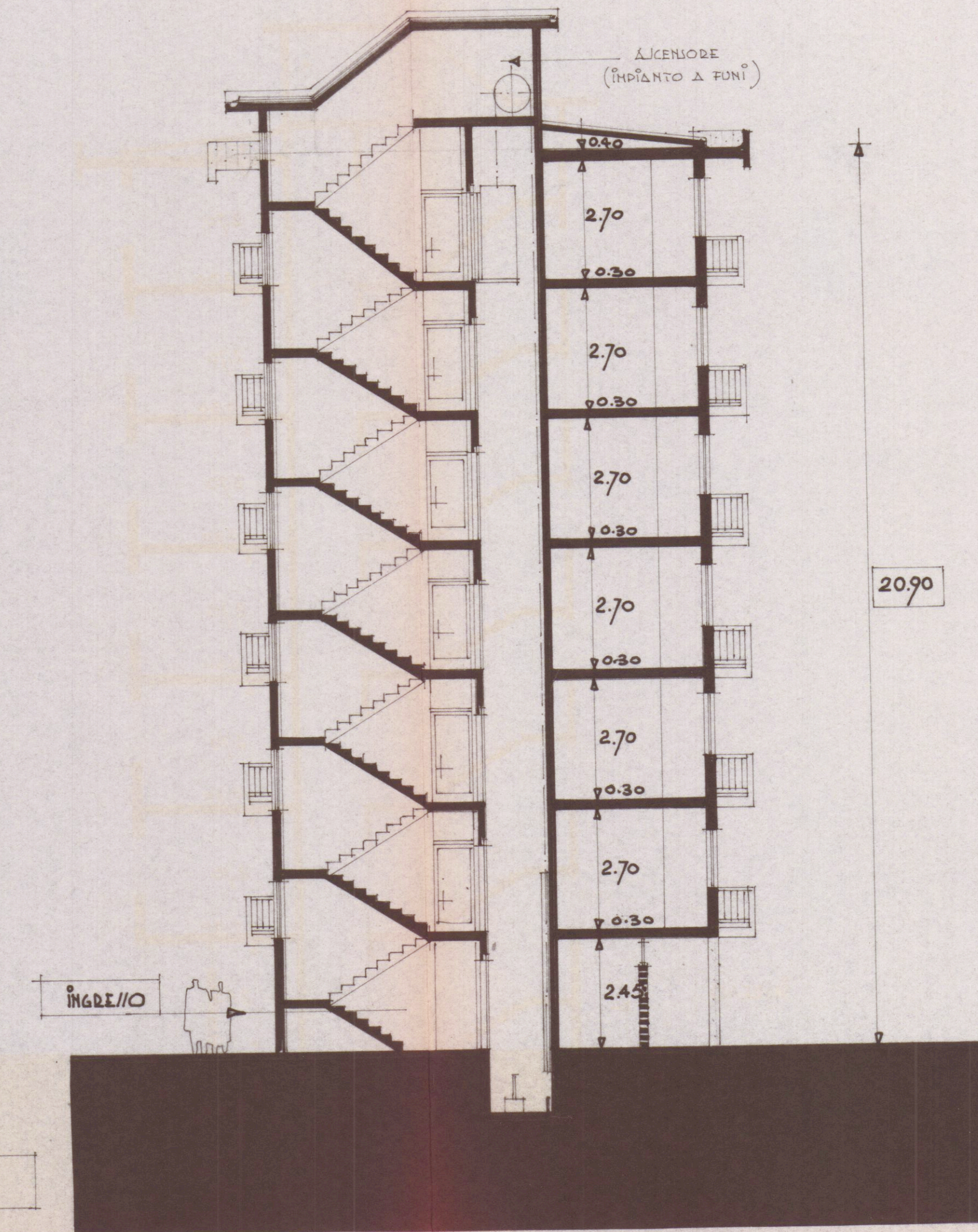
Sezione AB
