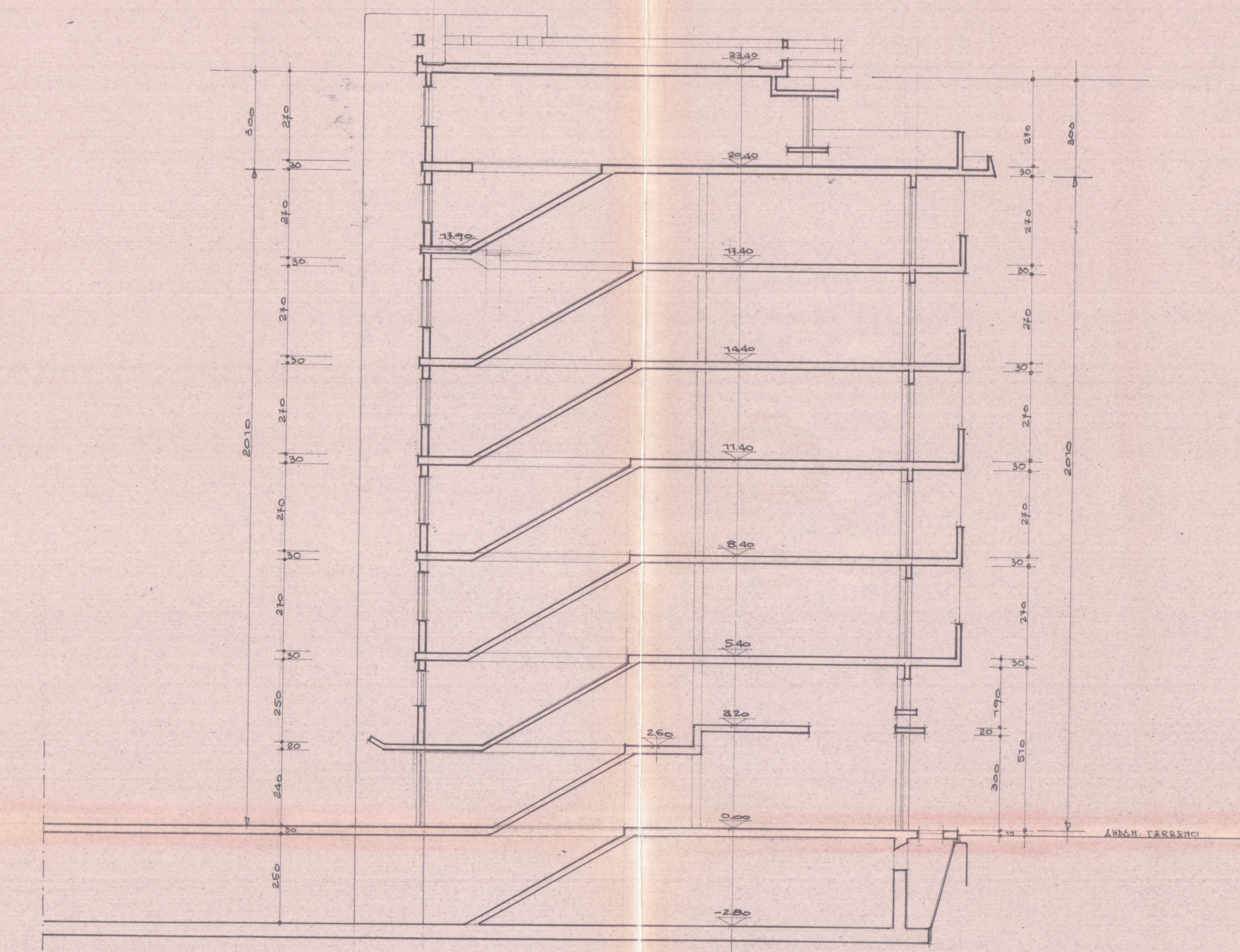
LEZIONE TRA/VER/ALE
