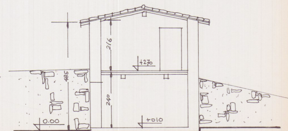
SEZIONE B-B
