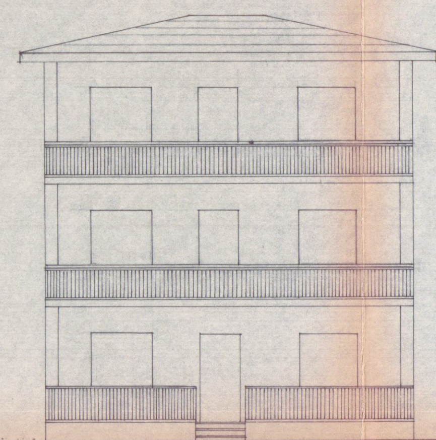
PROSPETTO VERSO VIA ADRONA
