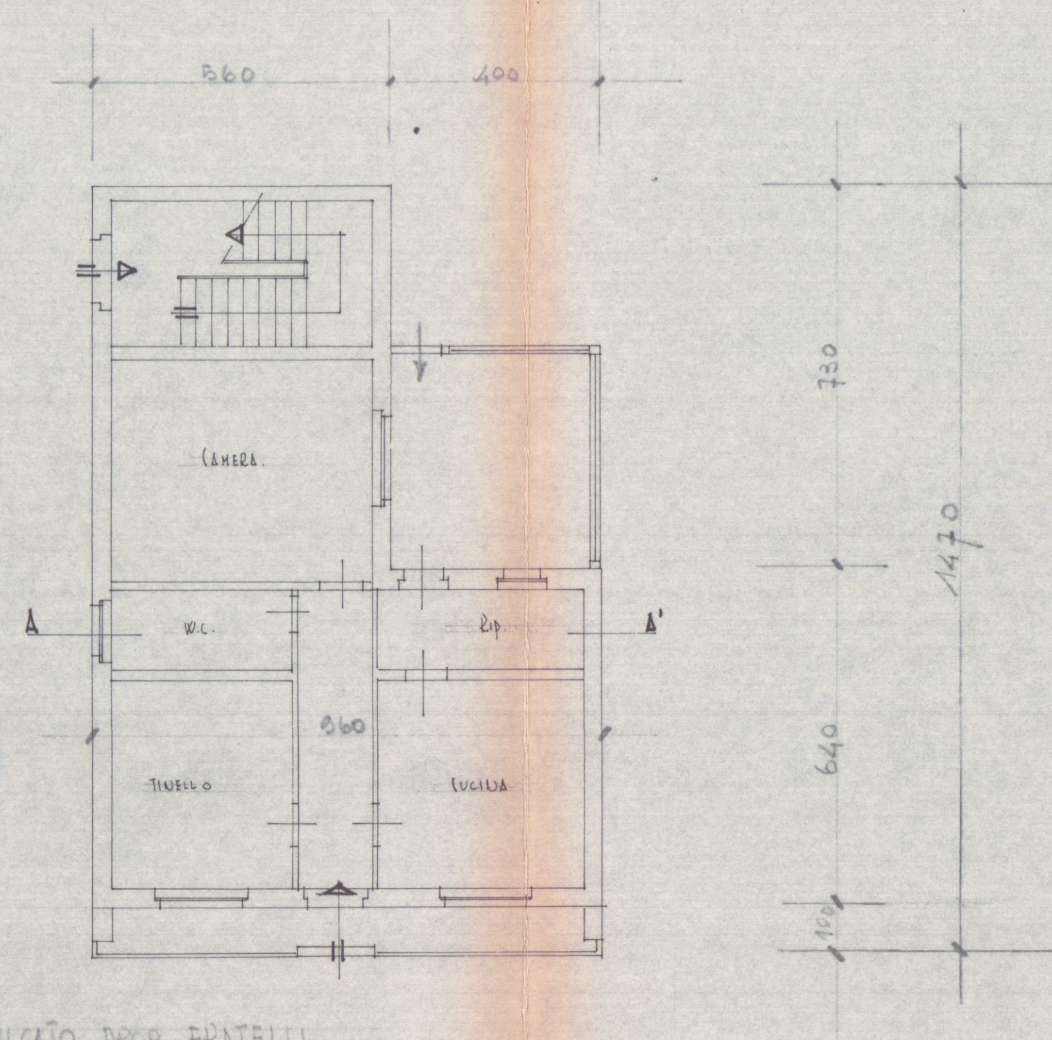
PIANO TERRA.
