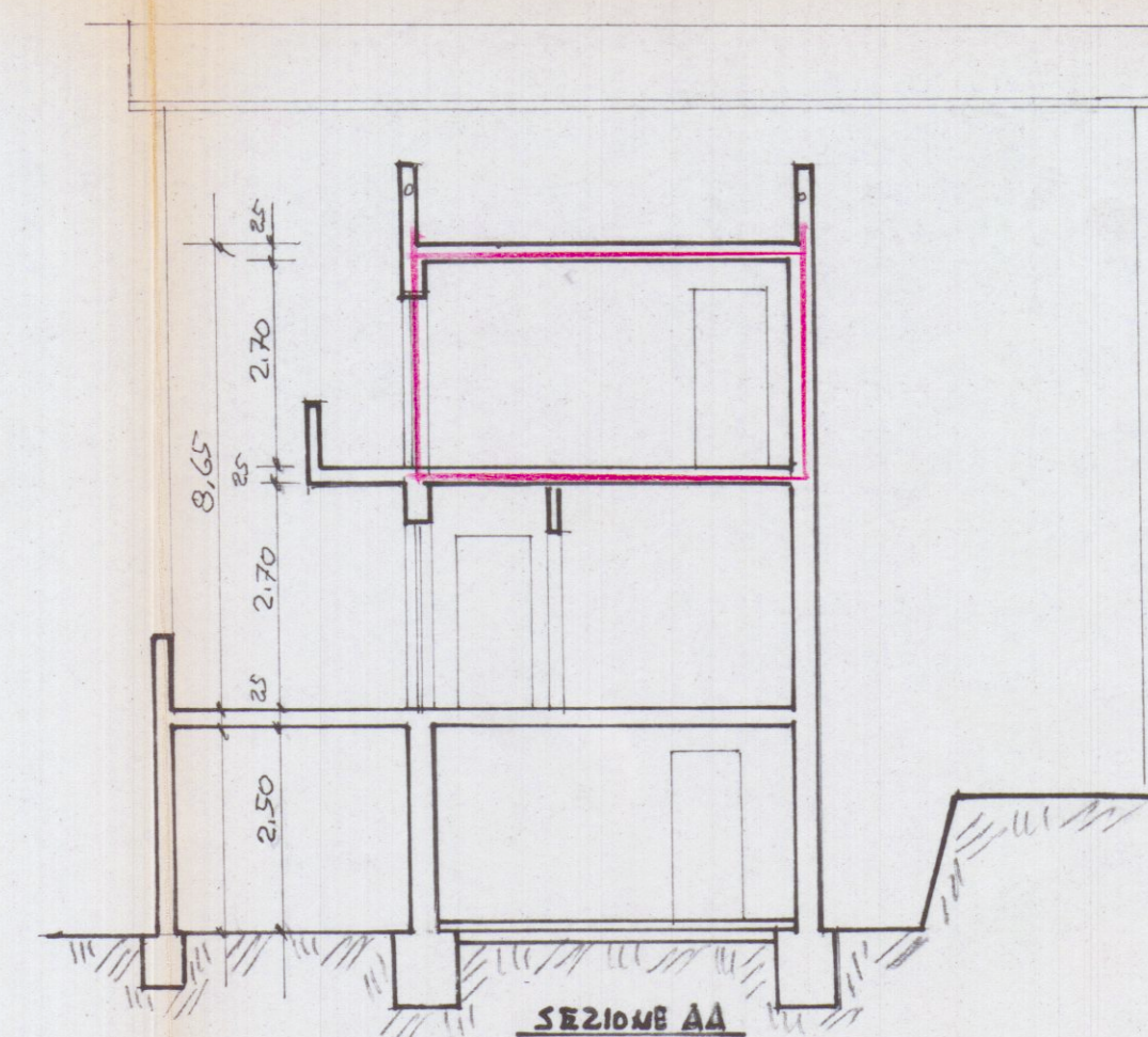
SEZIONE AA
