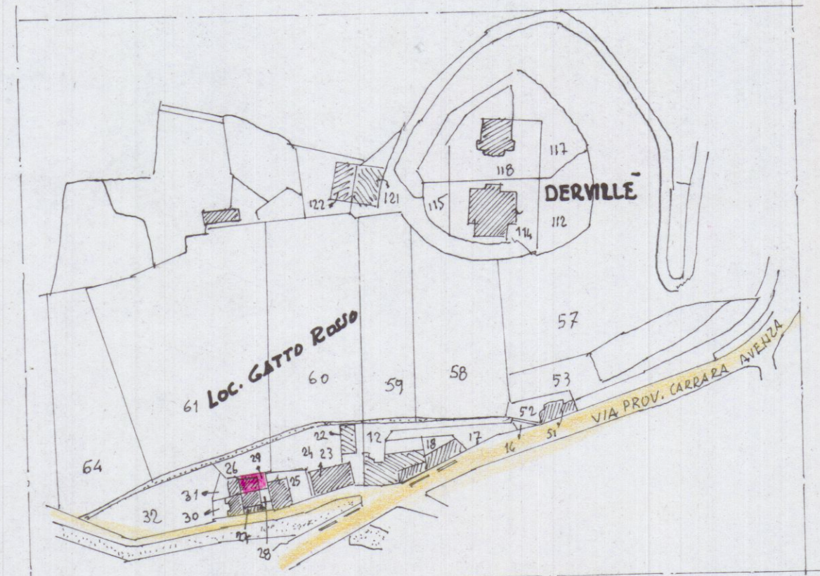
PLANIMETRIA 1/2000 - F. 66 MAPPOLE 29
