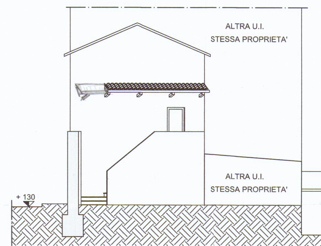
PROSPETTO OVEST
