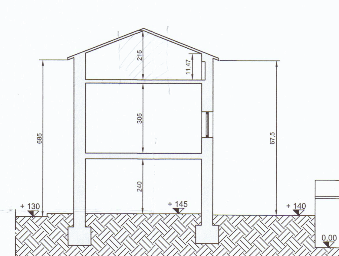
SEZIONE A-A
