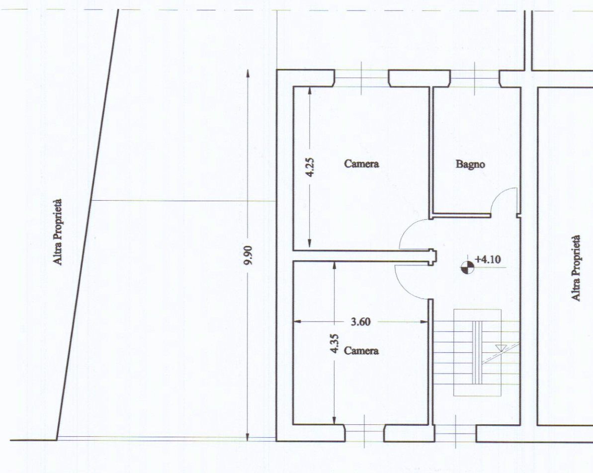
PIANTA PIANO PRIMO DI PROGETTO
