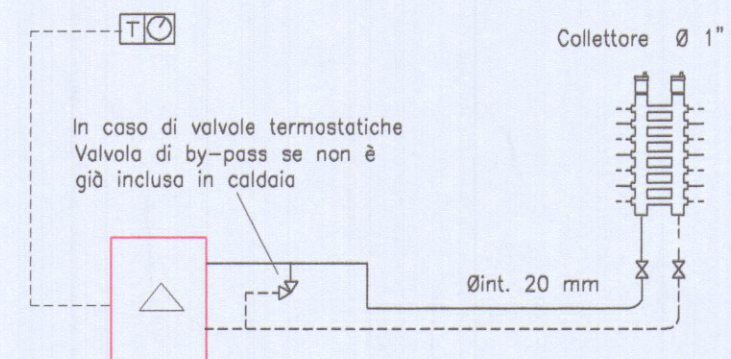
SCHEMA TIPO
