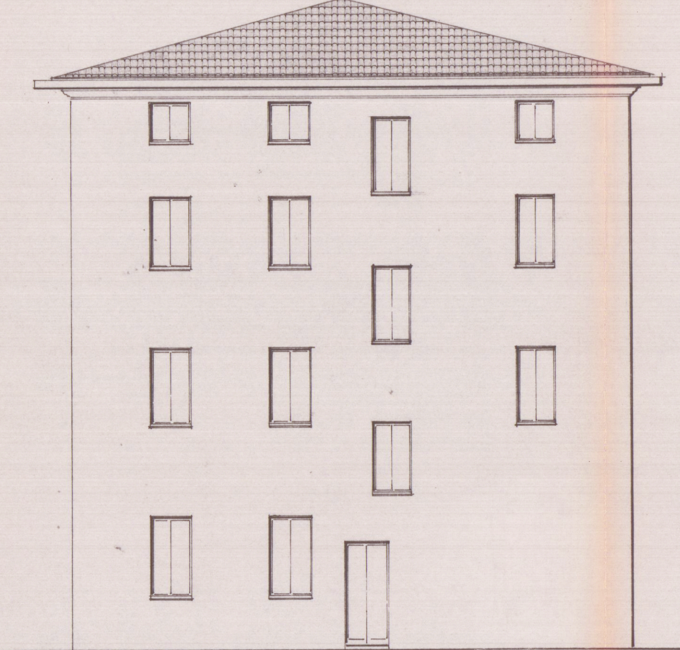
PROSPETTO NORD (SUL CORTILE)
