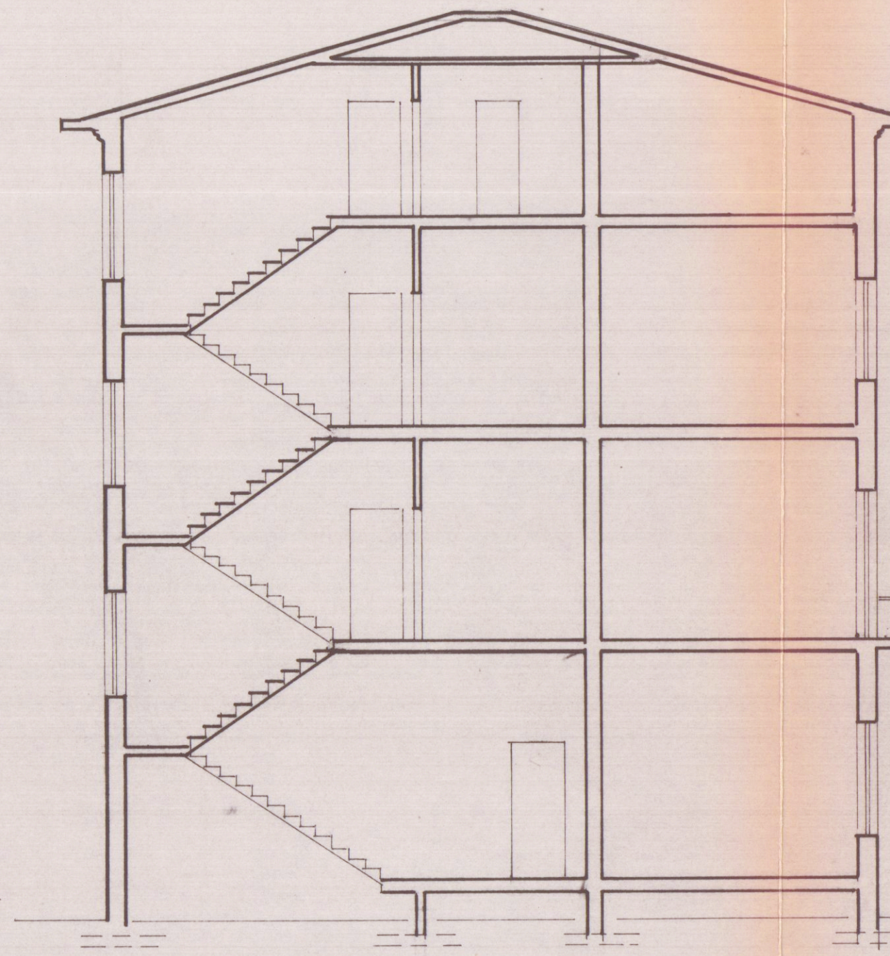
SEZIONE A-A'
