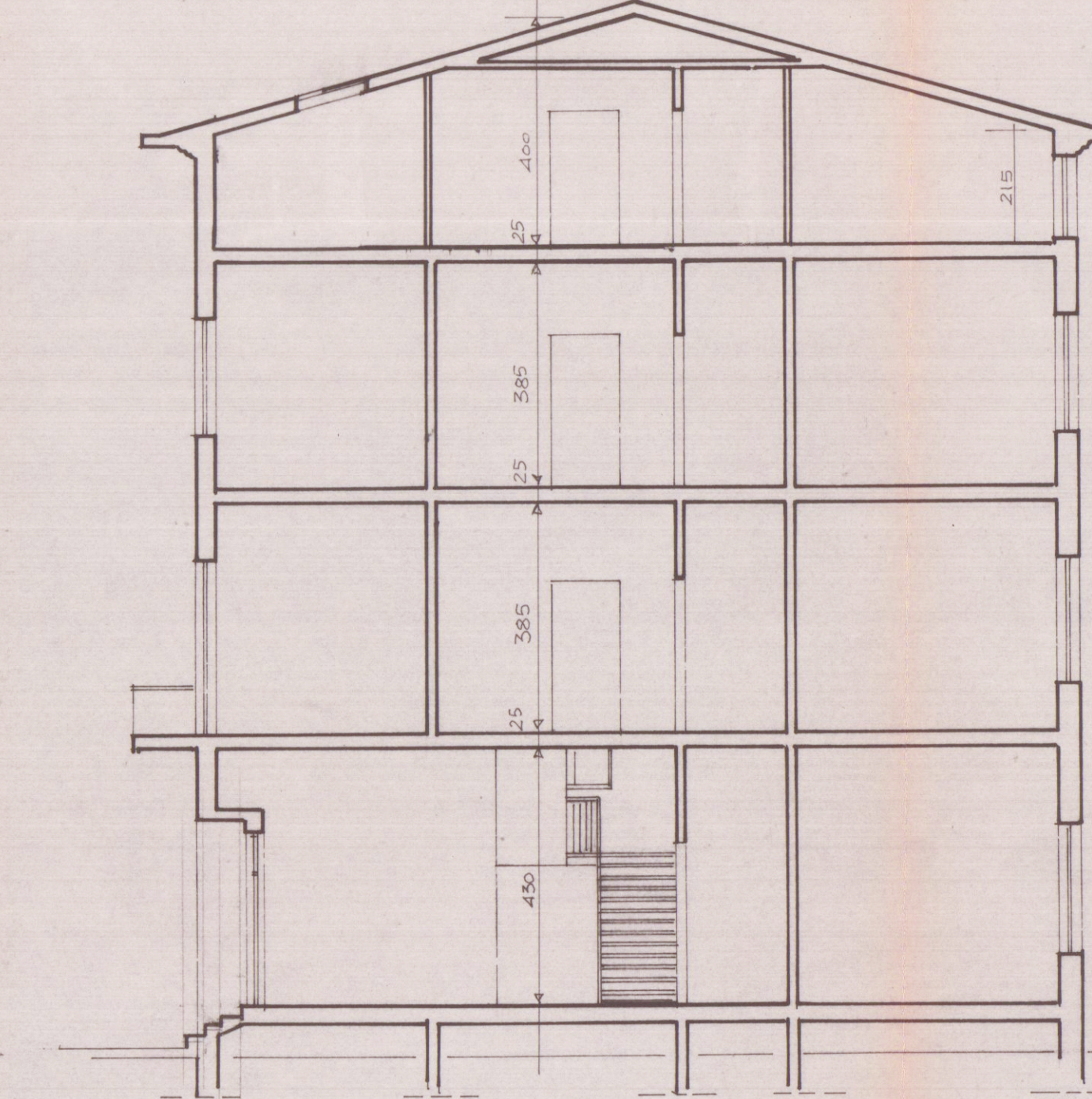
SEZIONE B-3
