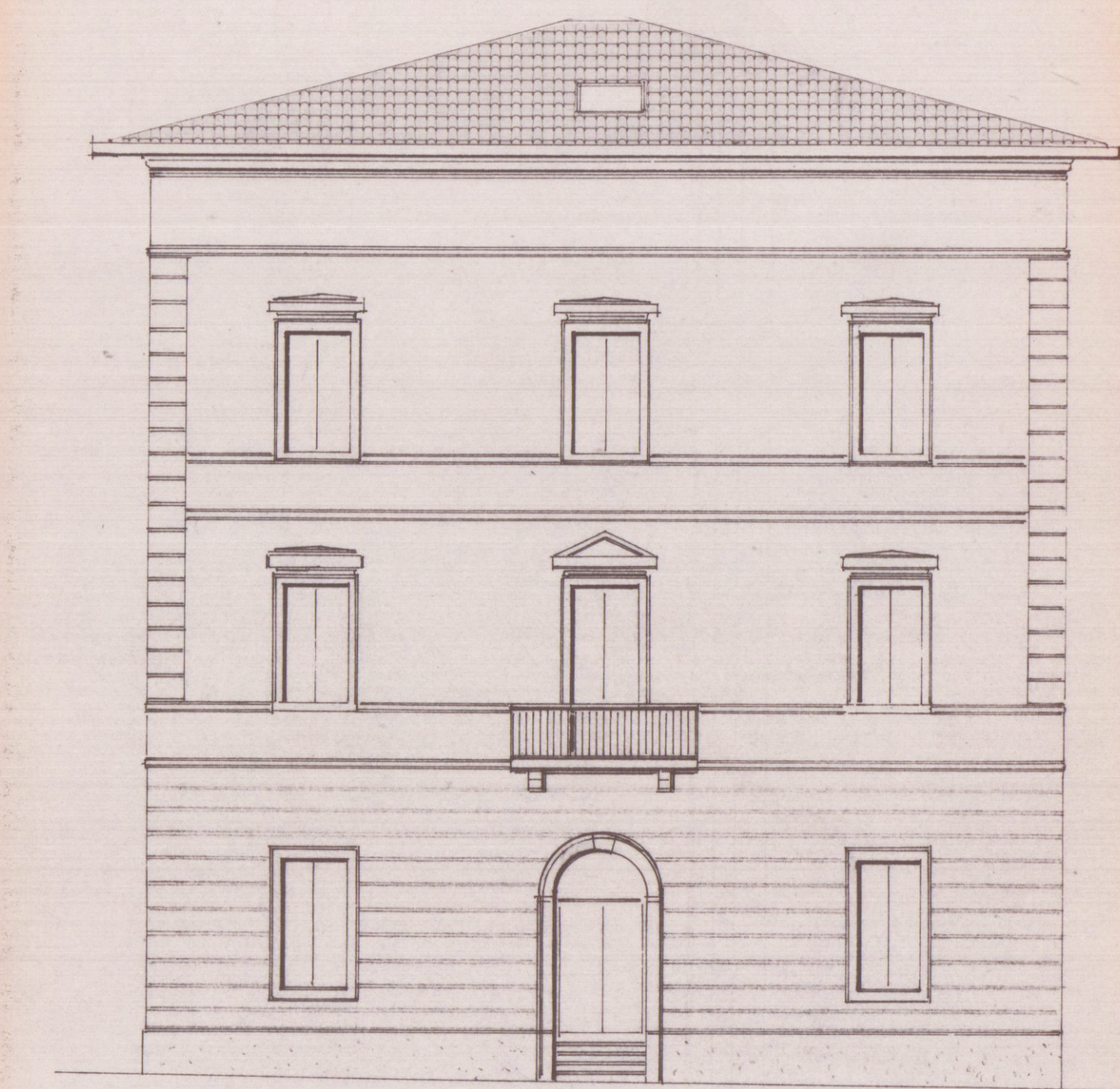
PROSPETTO SU V. CUCCHIARI
