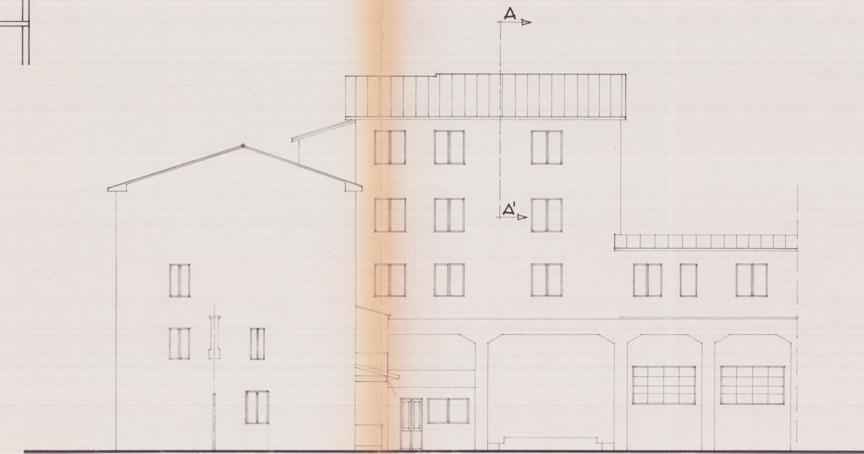
PROSPETTO NORD
