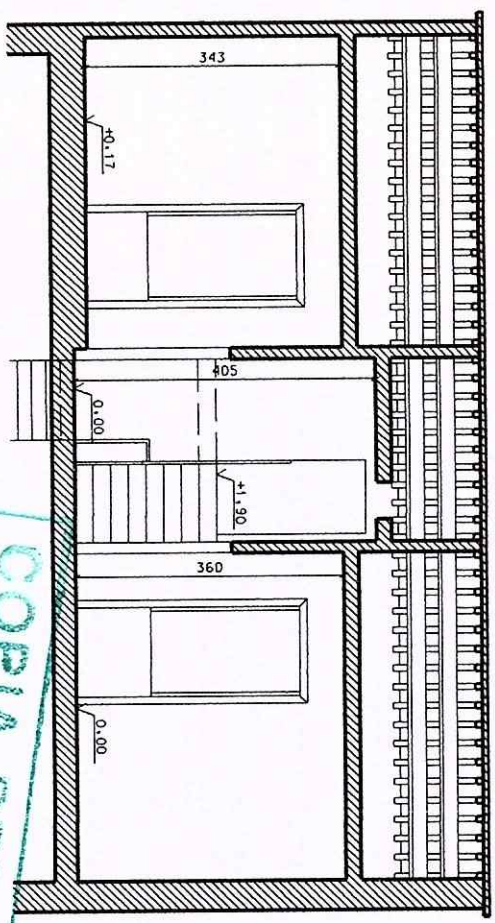
SEZIONE D
