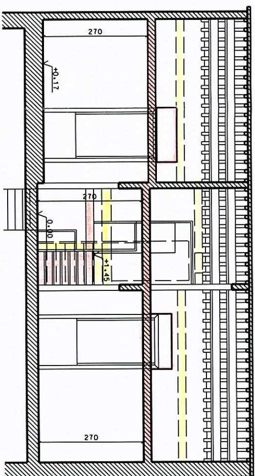
SEZIONE D
