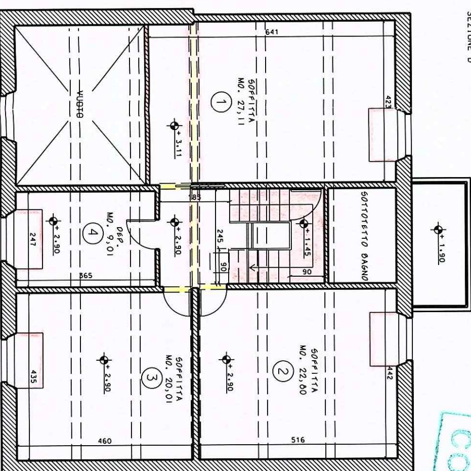
PIANTA SOTTOTETTO
