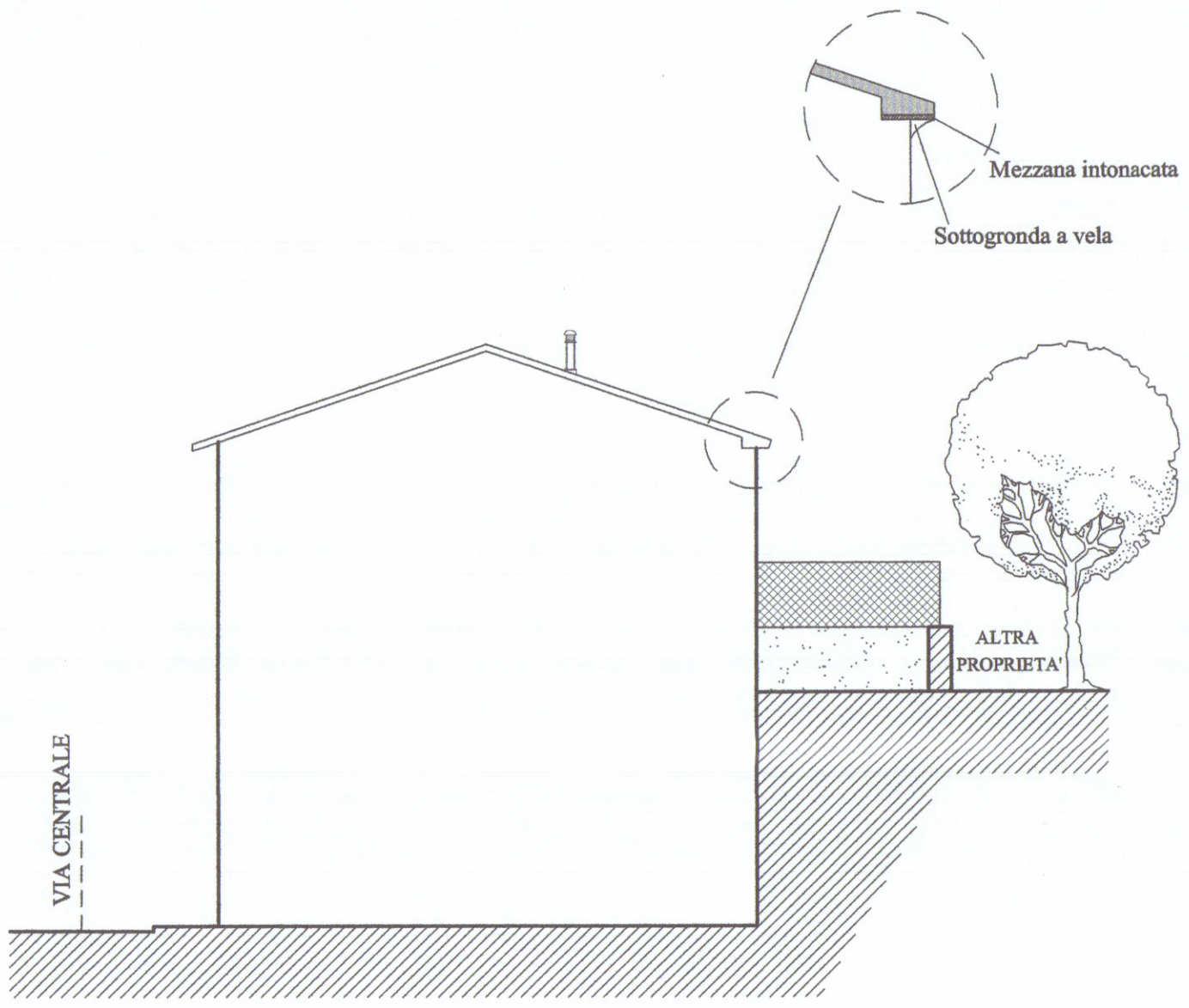
PROSPETTO INTERNO
