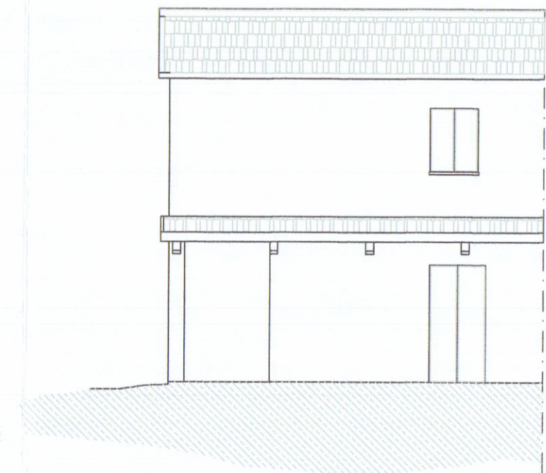
PROSPETTO LATERALE scala 1.100
