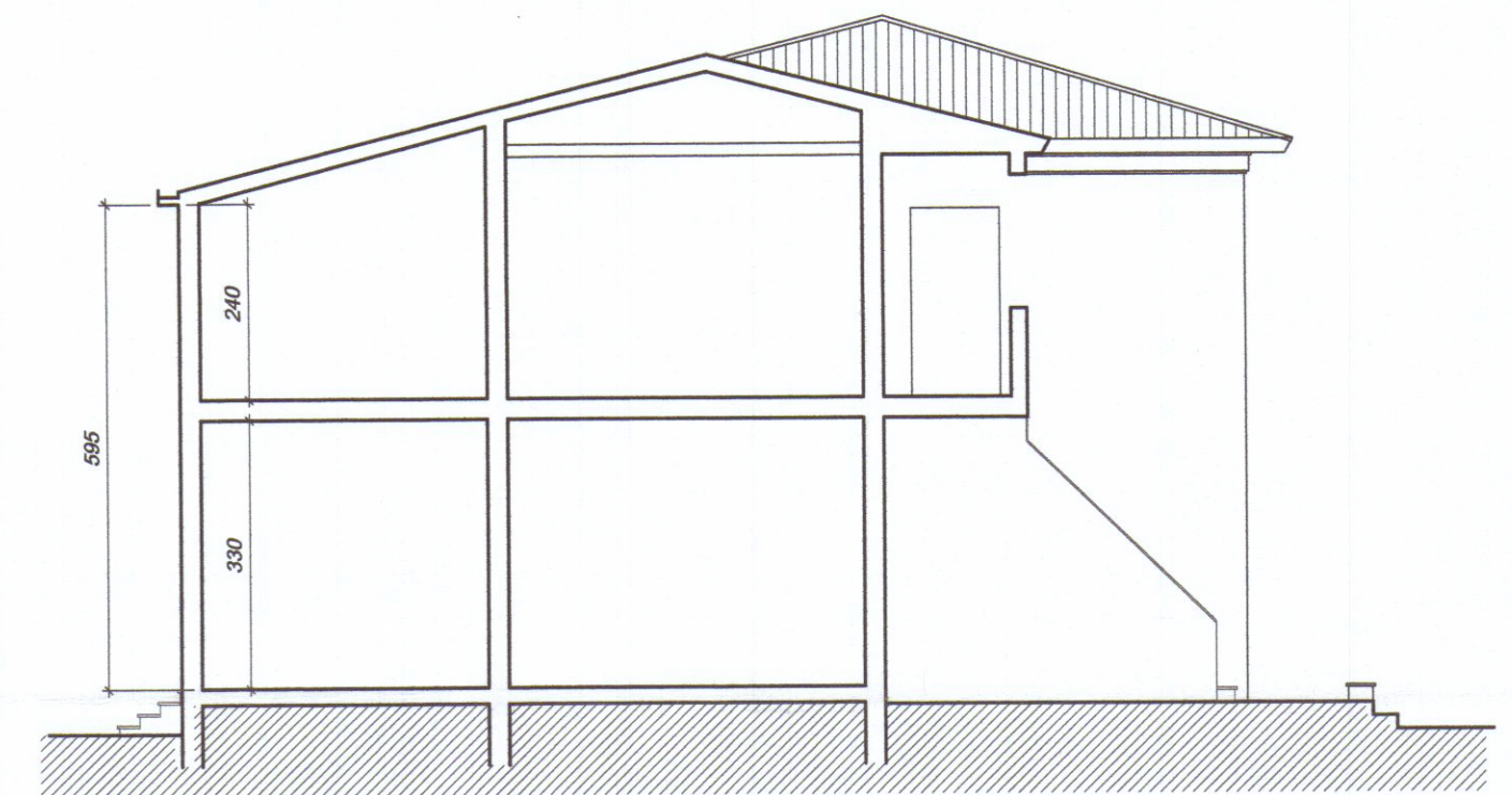
Sezione A-A
