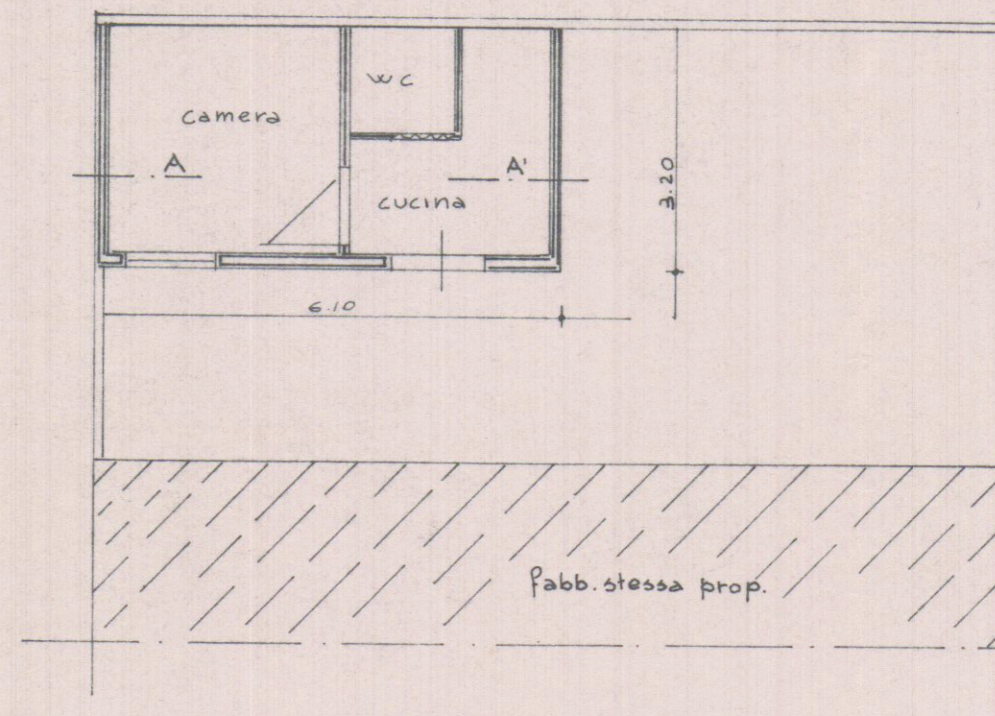
PIANTA
