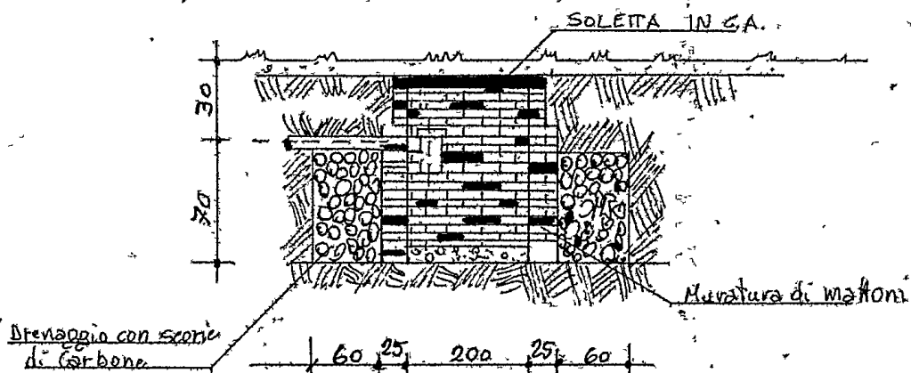
SEZIONE A-B
