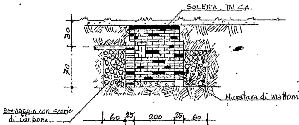
SEZIONE A-B
