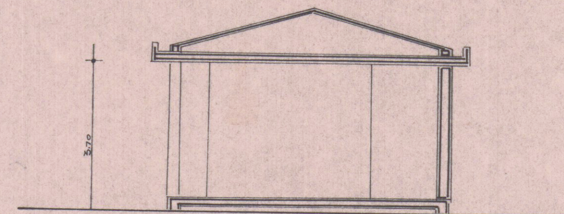
sezione AA realizzata
