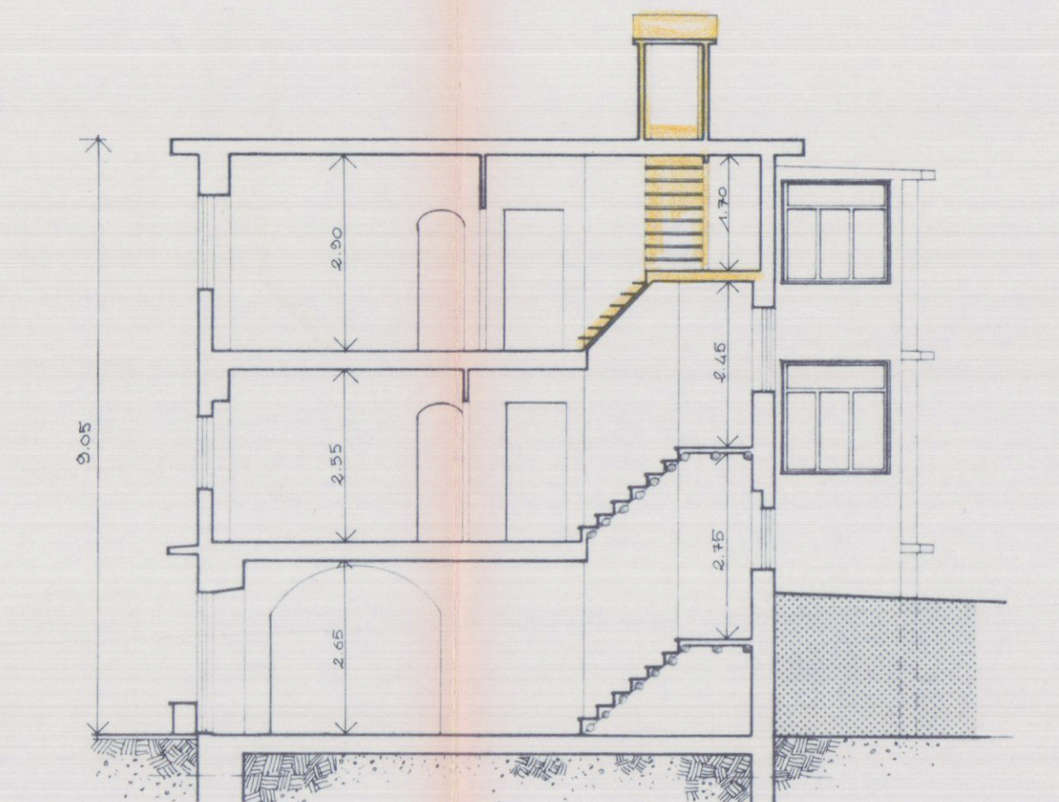
SEZIONE B-B'
