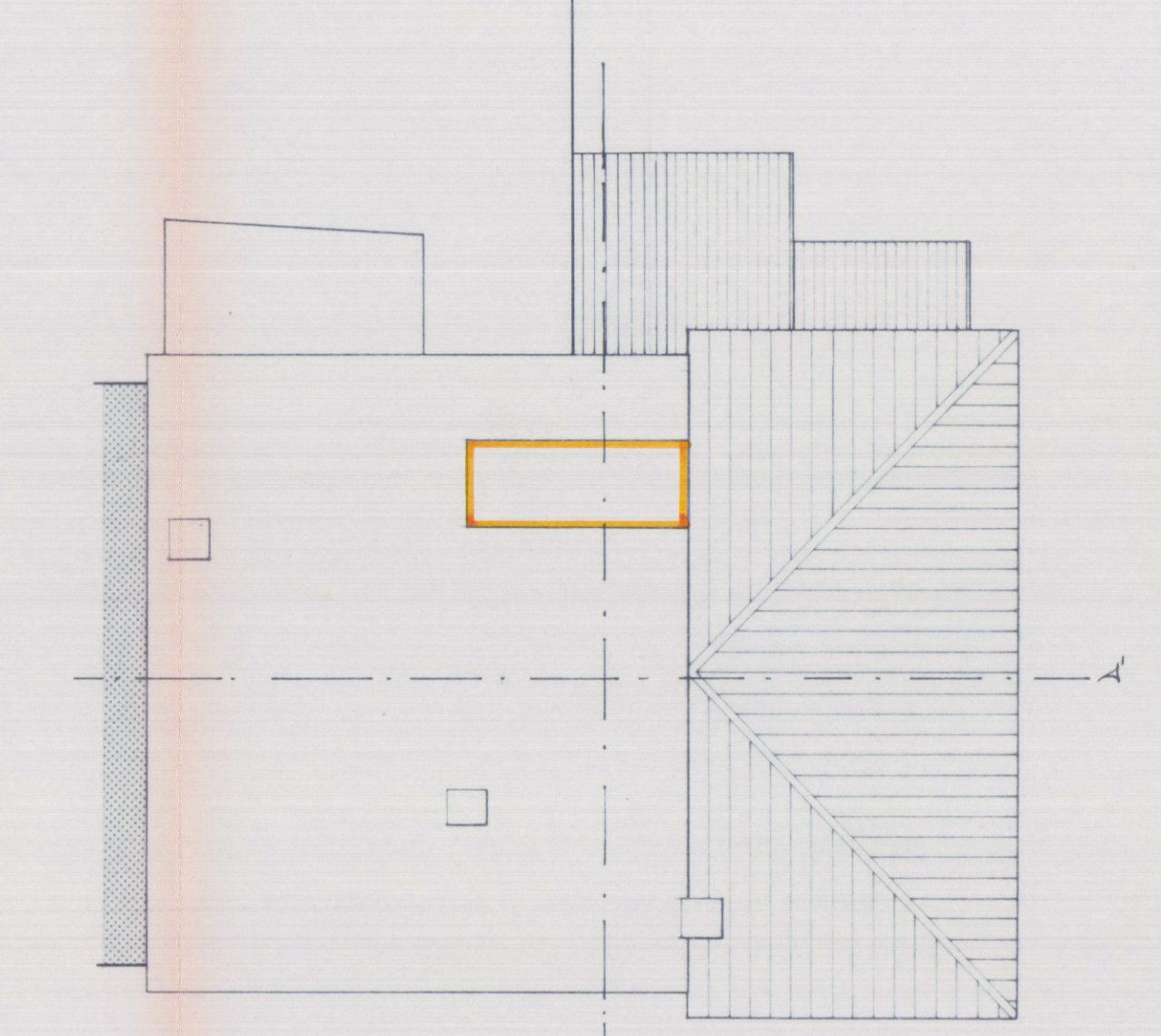
PIANTA COPERTURA
