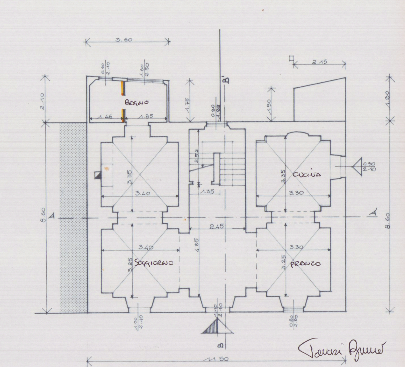
PIANTA DIAMO TERRA
