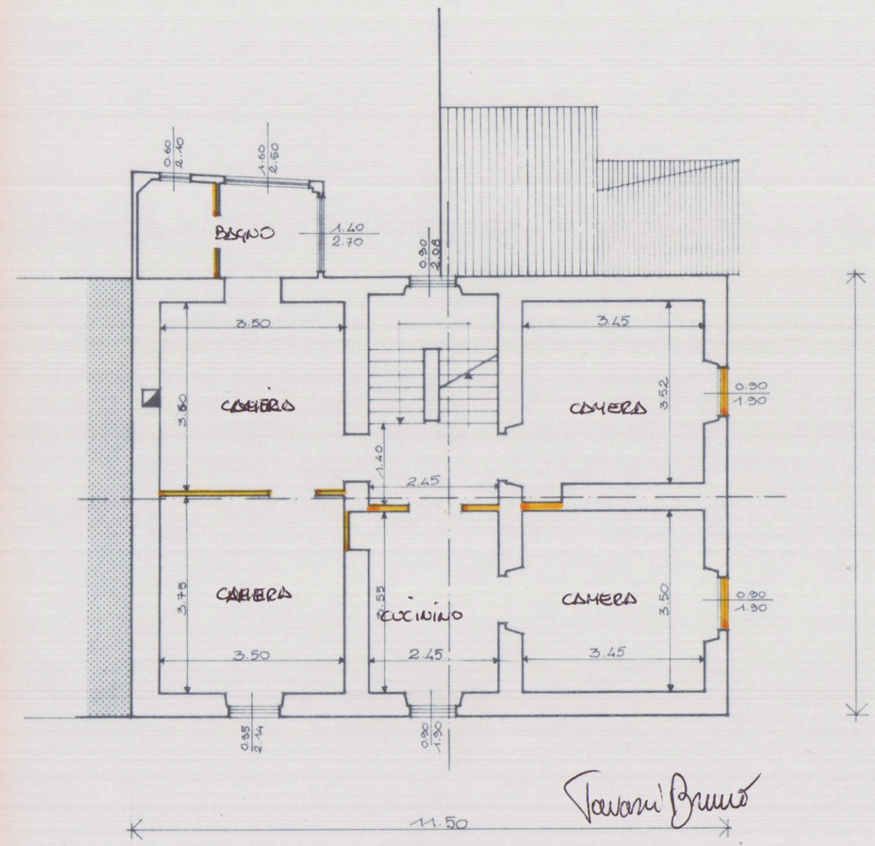
PIANTA DIAMO PRIMO
