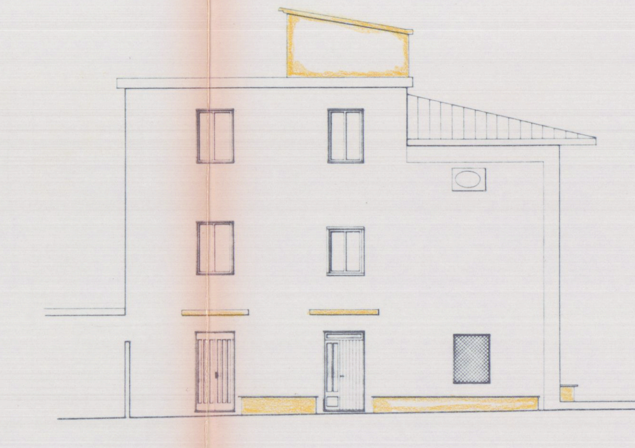
PROSPETTO SUD
