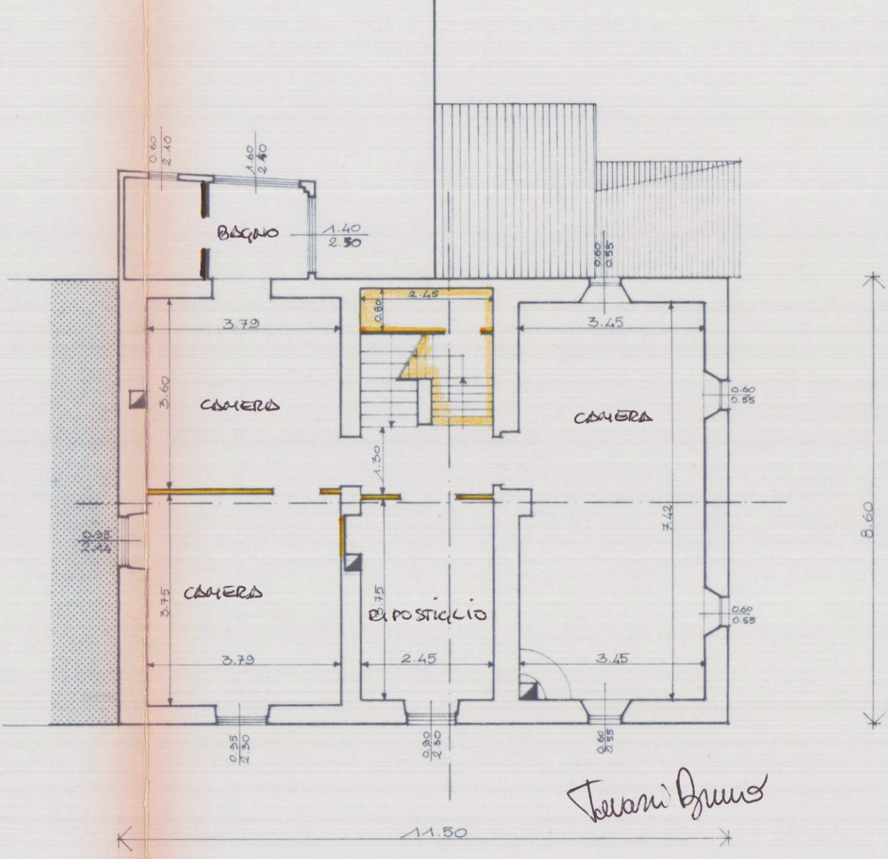
PIANTA DIAMO SECONDO
