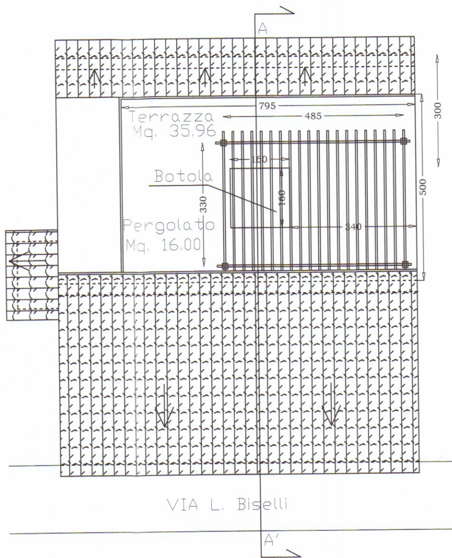
Pianta Copertura
