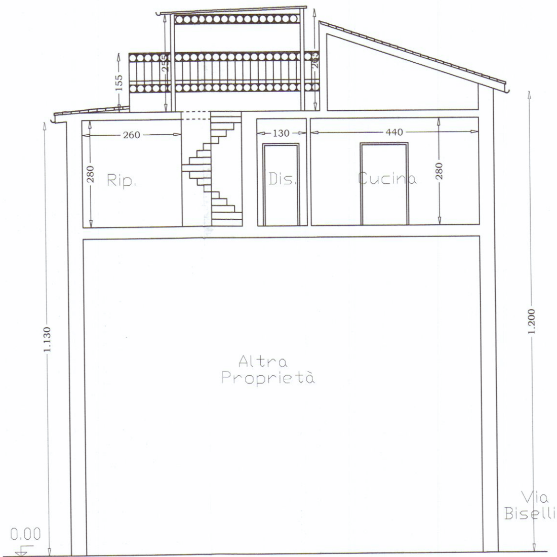
Sezione A-A'
