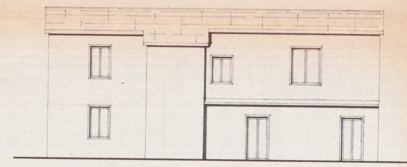
PROSPETTO SUB MODIFICATO
