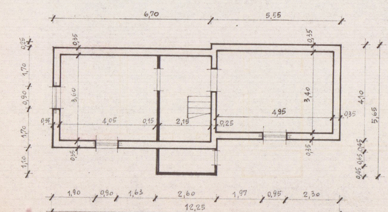
PIANTA PIANO TERRA ESISTENTE
