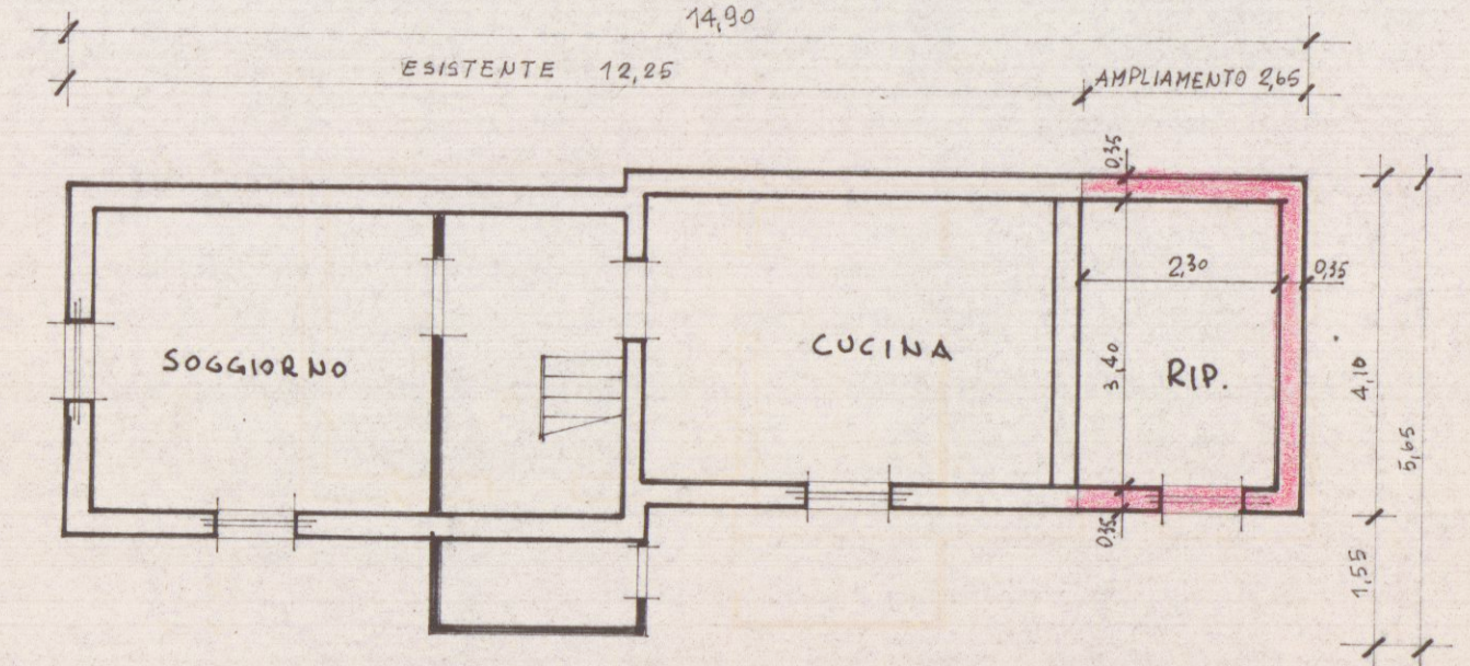
PIANTA PIANO TERRA AMPLIATO
