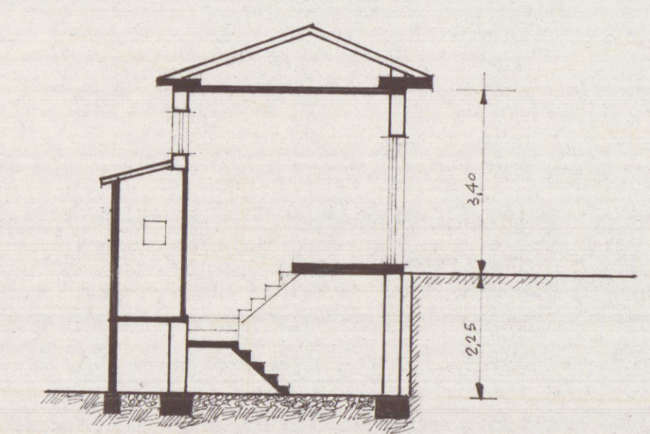
SEZIONE A-A ESISTENTE
