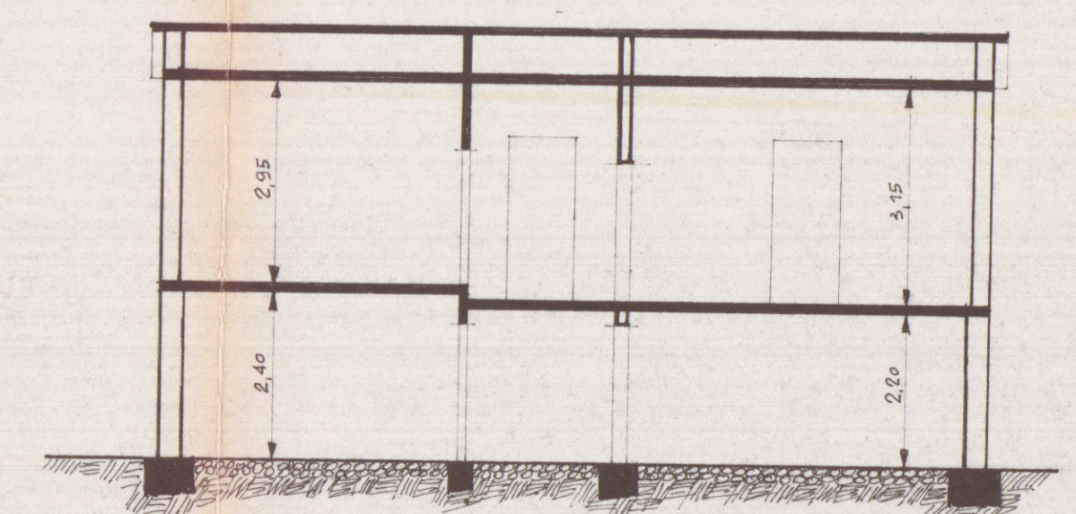
SEZIONE B-B ESISTENTE
