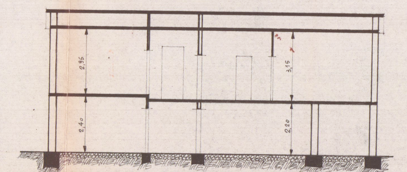
SEZIONE B-B MODIFICATA
