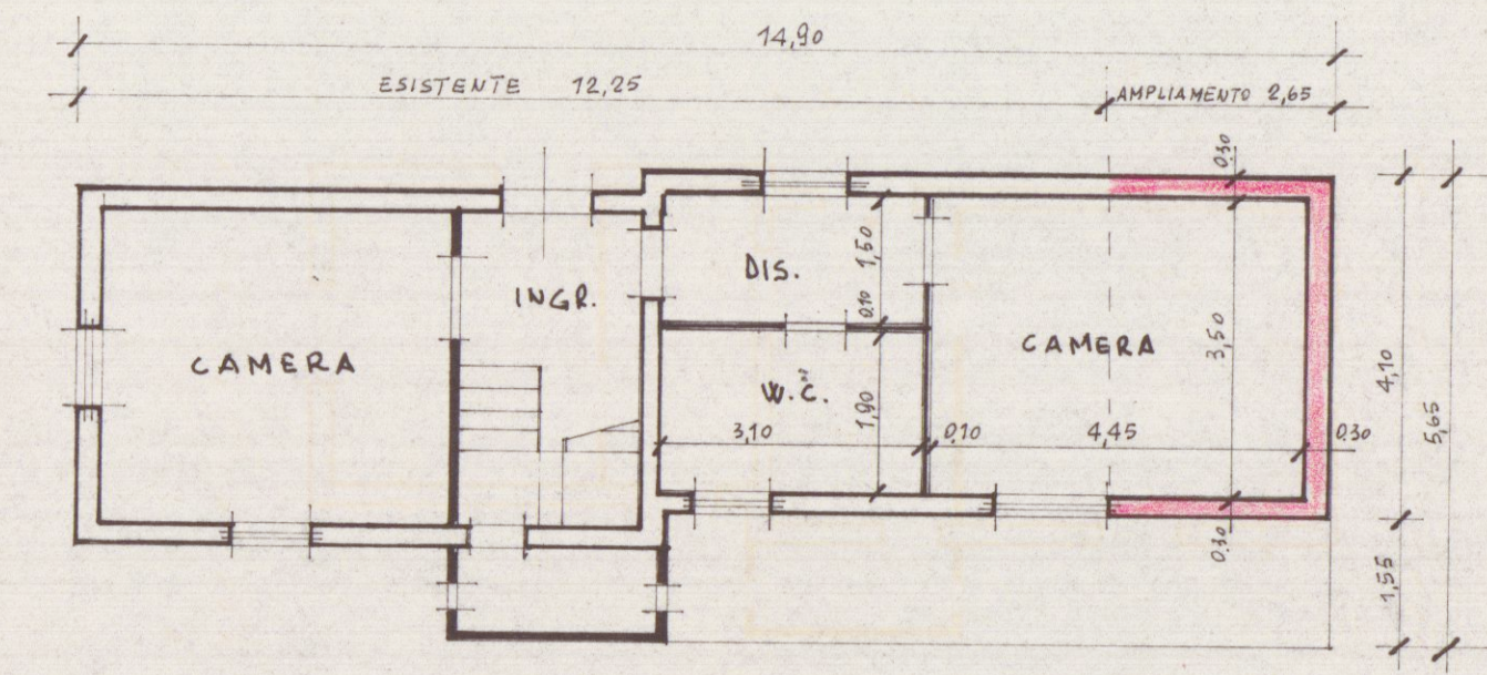
PIANTA PRIMO PIANO AMPLIATO
