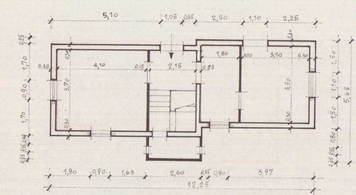
PIANTA PRIMO PIANO ESISTENTE
