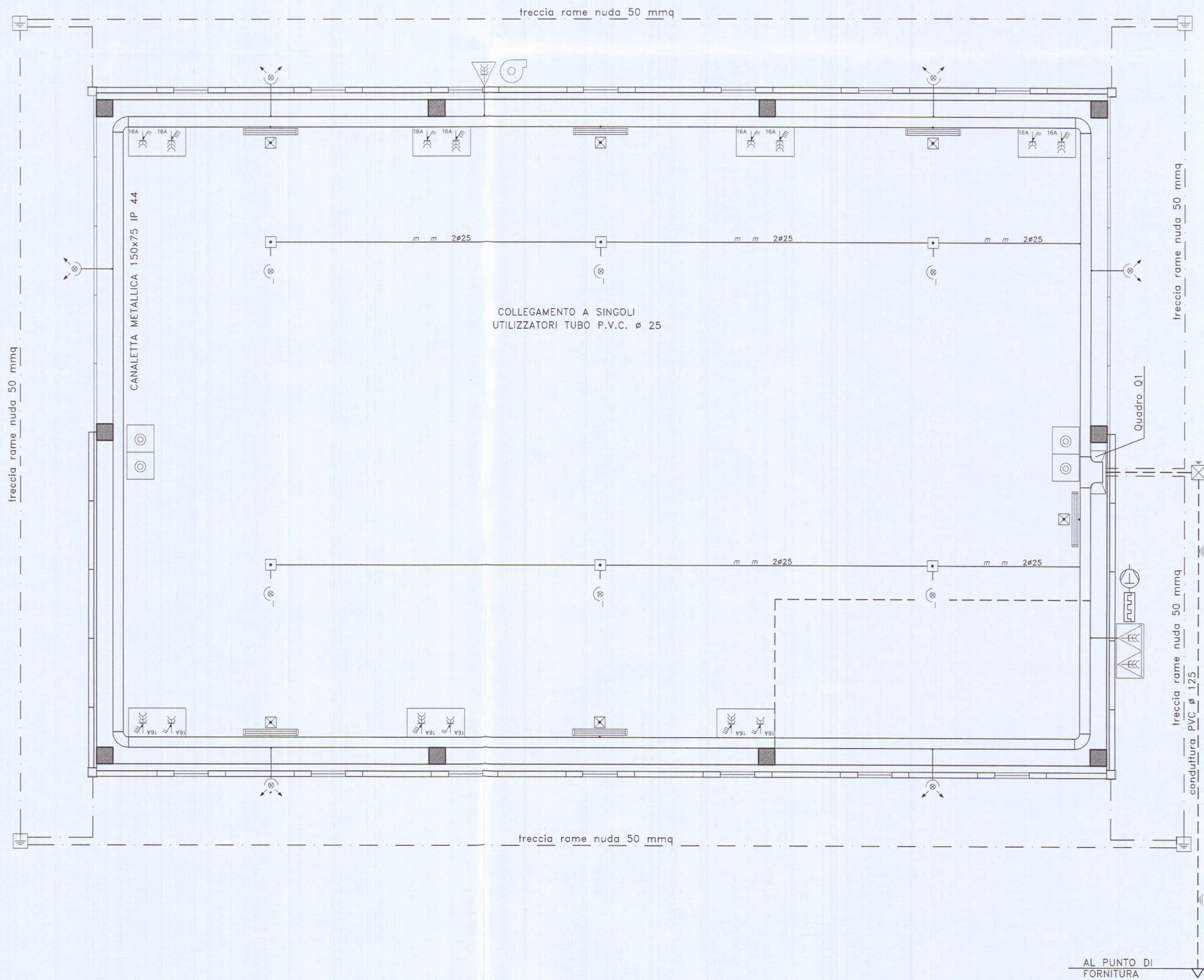
PIANTA LABORATORIO
