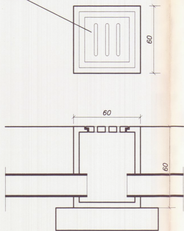
POZZETTO PER FOGNATURA STRADALE
