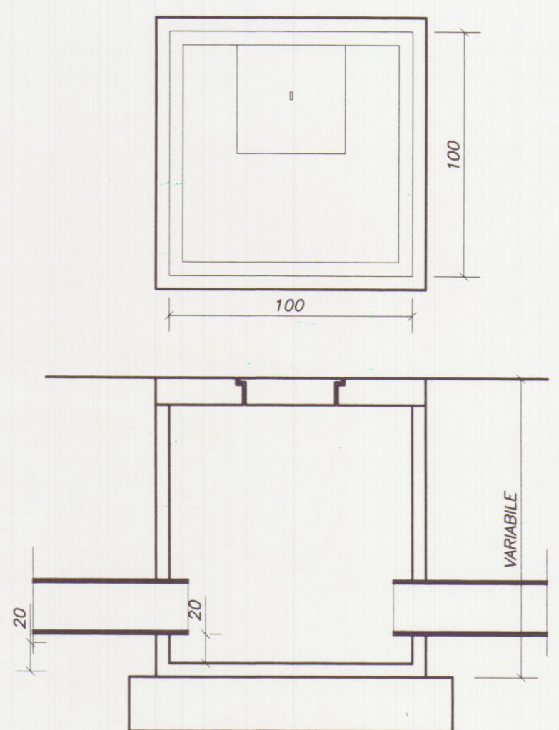
POZZETTO DI ISPEZIONE ACQUE BIANCHE
