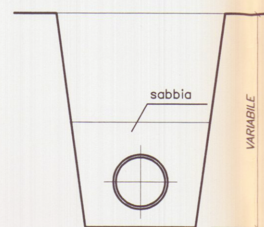
SCAVO TIPO ACQUE NERE
