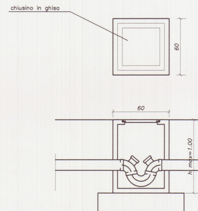
POZZETTO DI ALLACCIO
