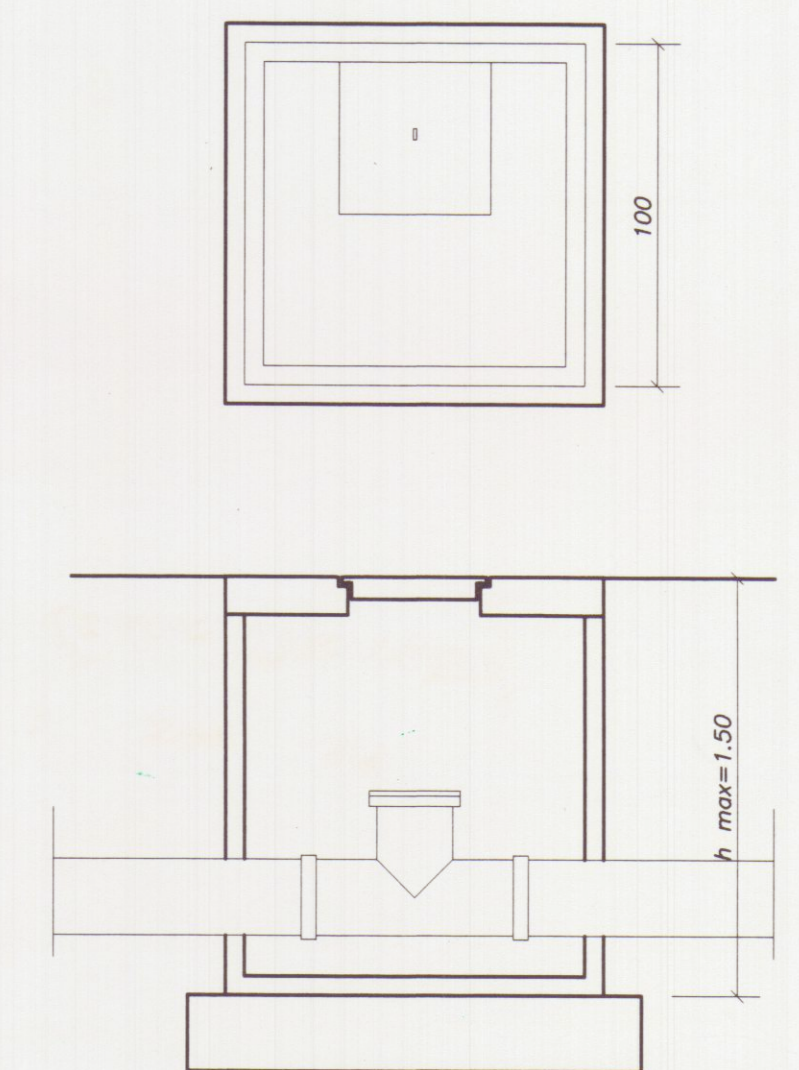
POZZETTO DI ISPEZIONE ACQUE NERE
