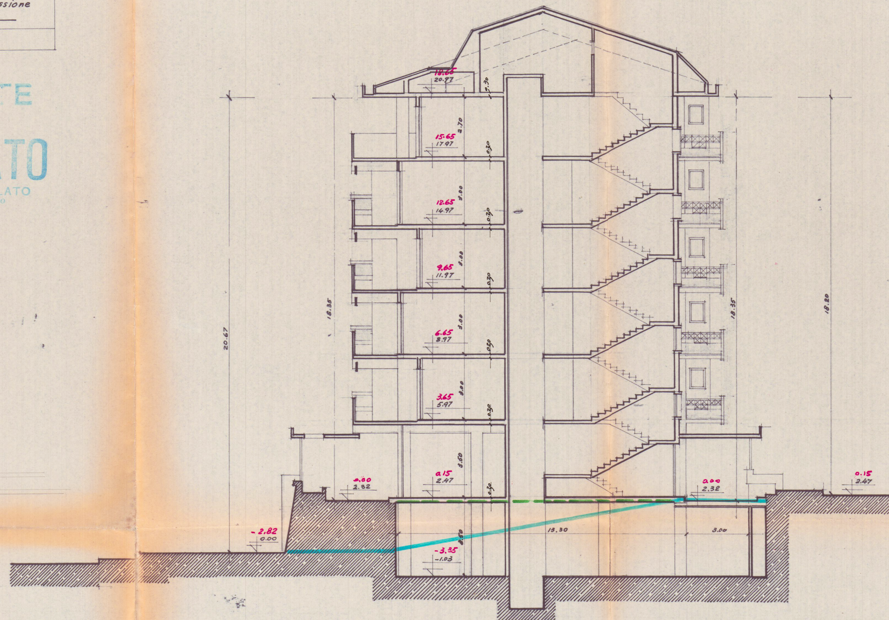
sezione AB
