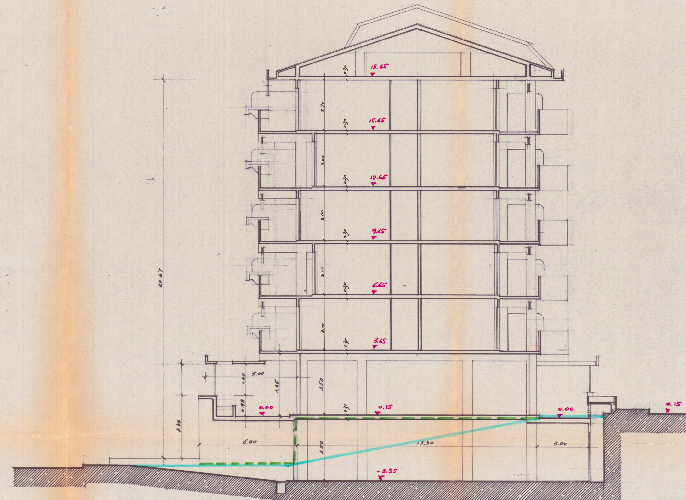
sezione CD
