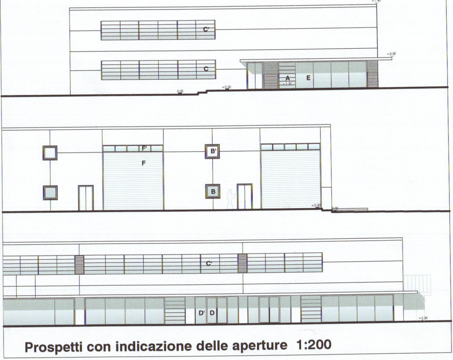
Prospecti con indicazione delle aperture 1:200
