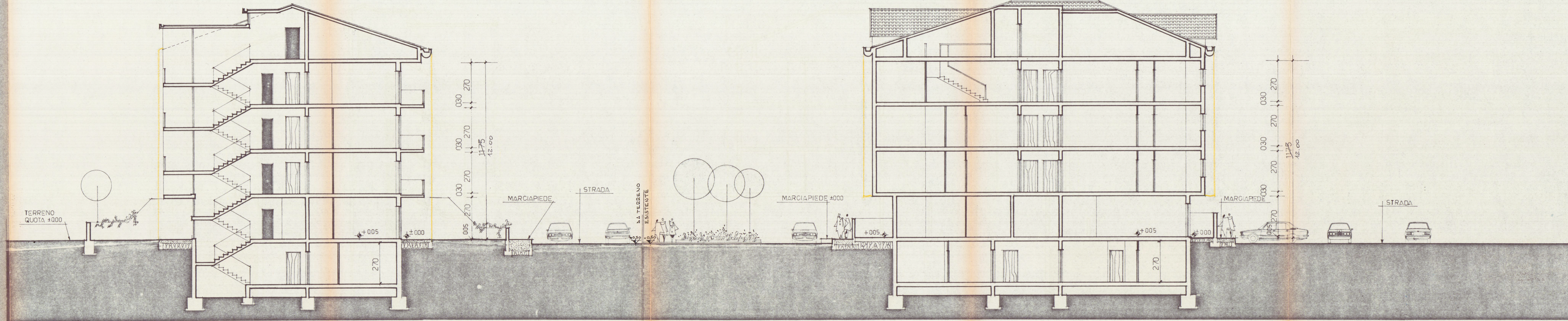
sezione a:a 1
