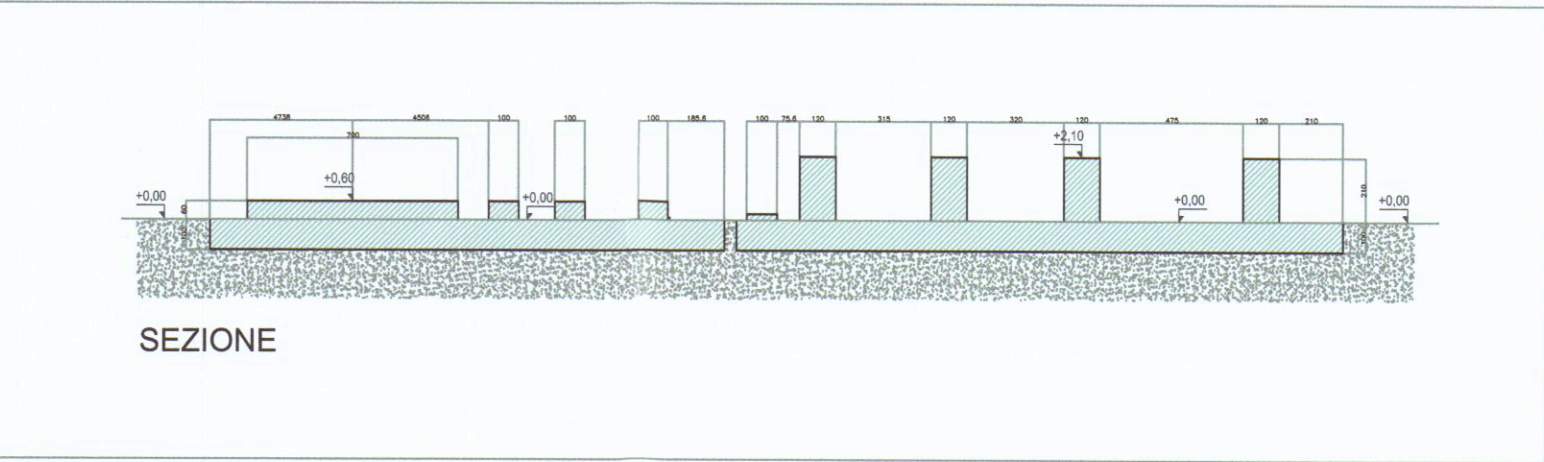
SEZIONE TIPOLOGICA PLATEE
