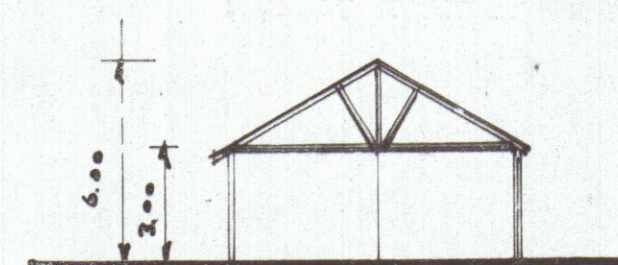
SEZIONE A-A
