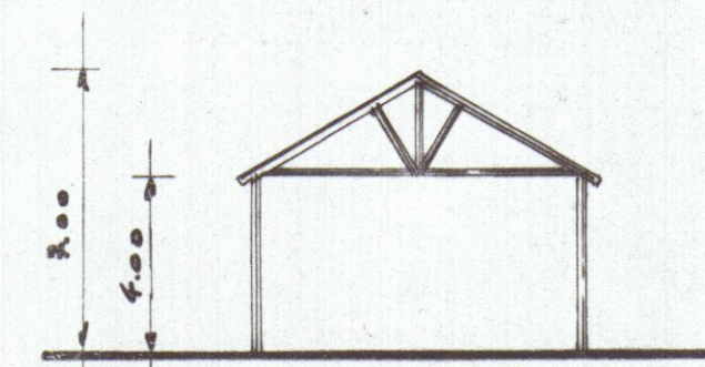
SEZIONE B-B
