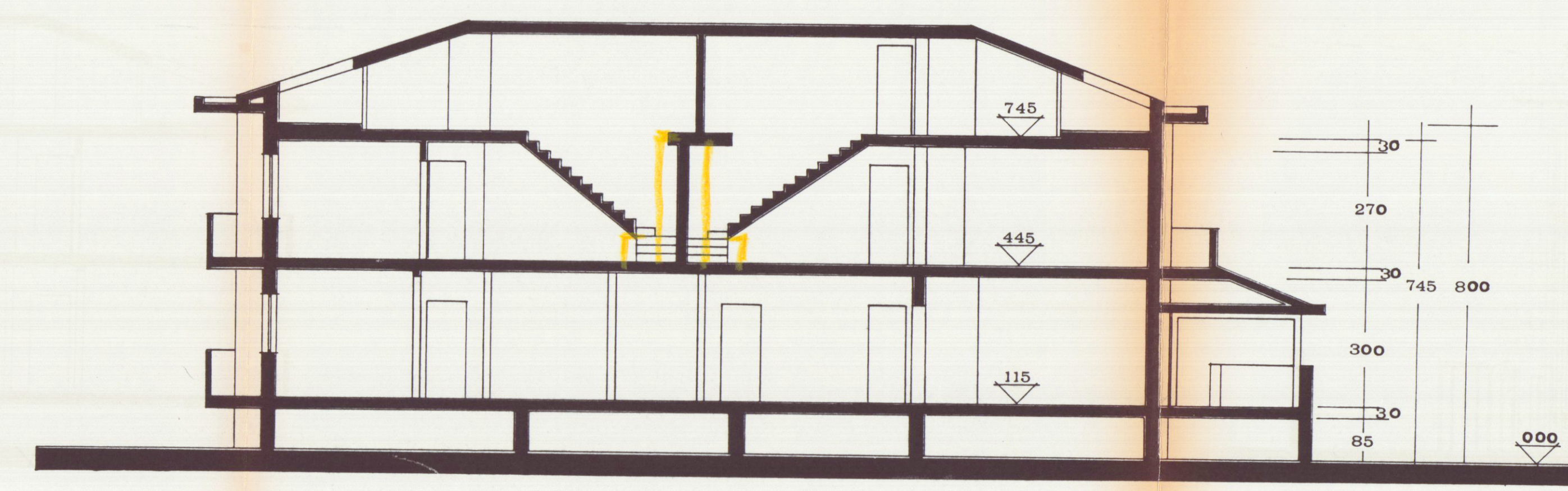
sez. A-A'
