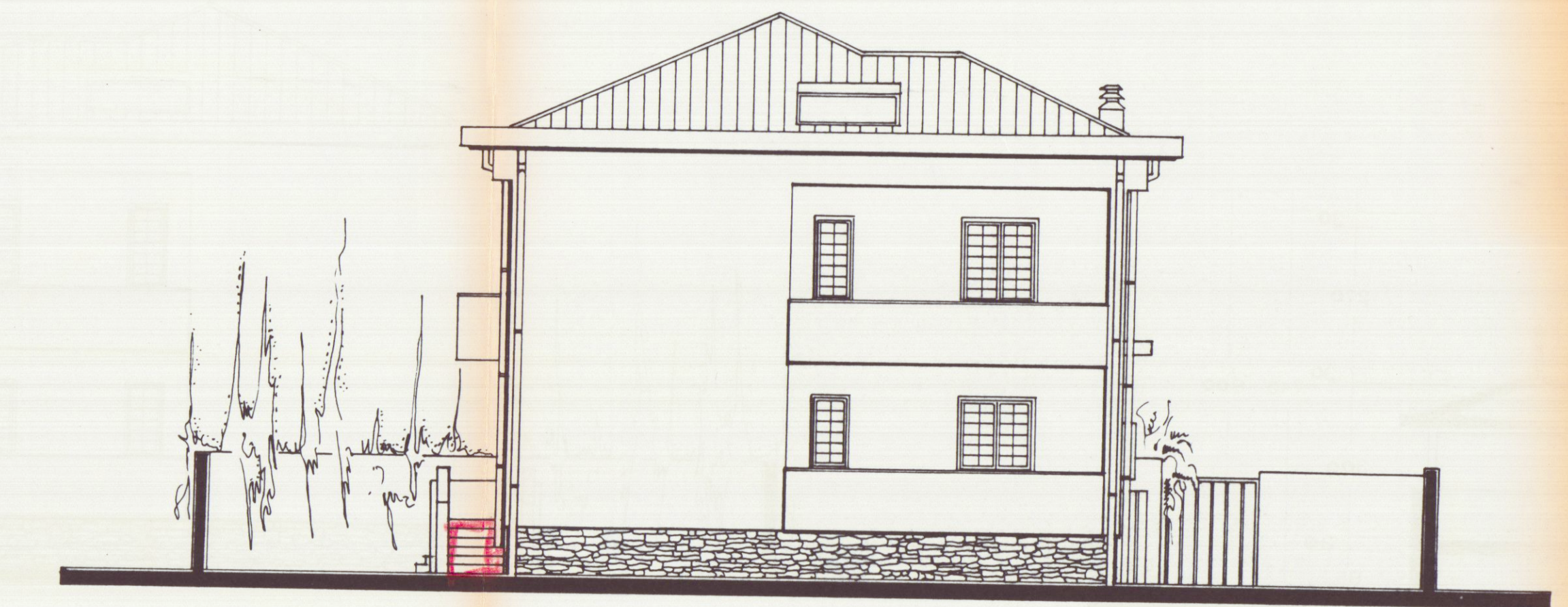
prospetto est
