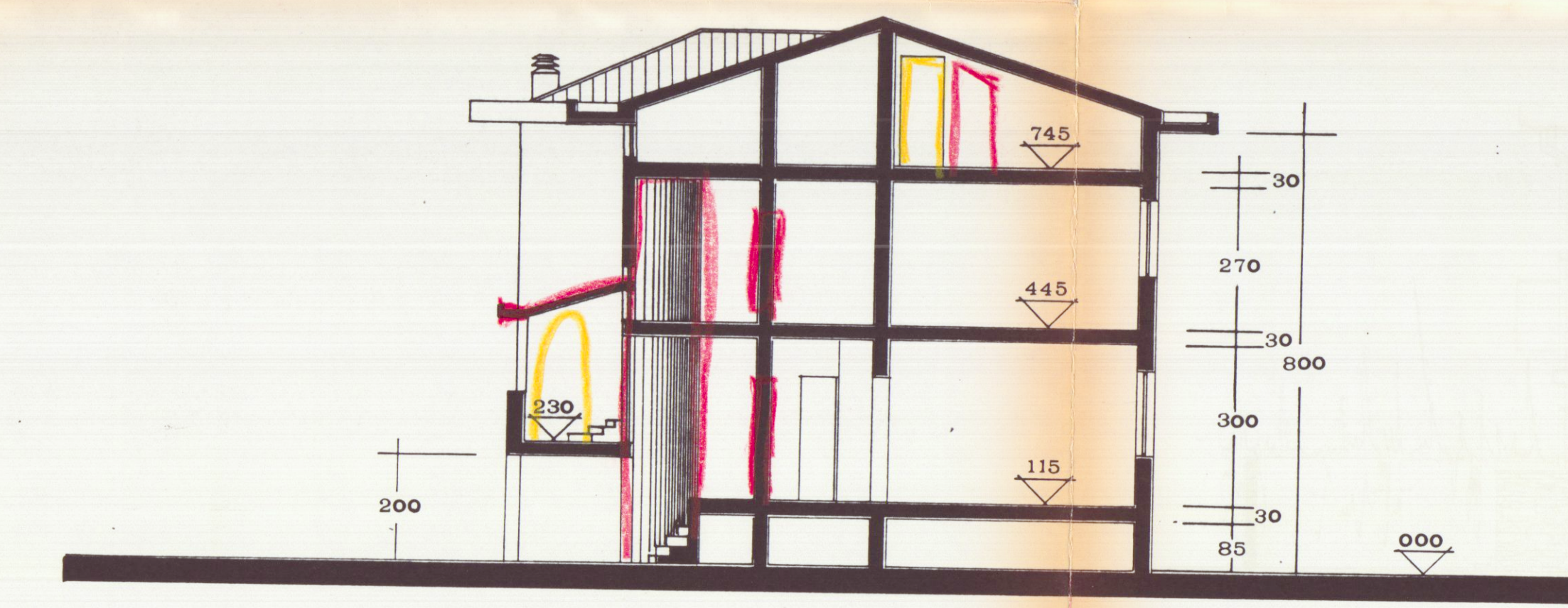
sez. B-B'
