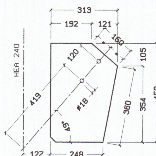
Lam. 120/10 P5 Costruire n° 2
