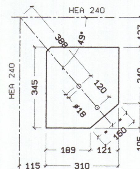
Lam.120/10 P6 Costruirne n° 2
