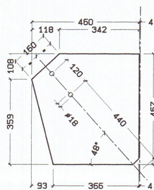
Lam.120/10 Pg Costruirne n° 1
