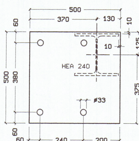
Lam. 300/10 P1A Costruirne n° 2
