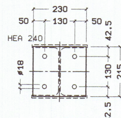
Lam. 120/10 P2 Costruime n° 9
