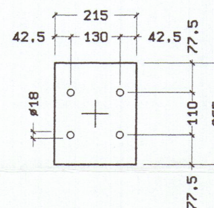
Lam. 120/10 P11 Costruire n° 2
