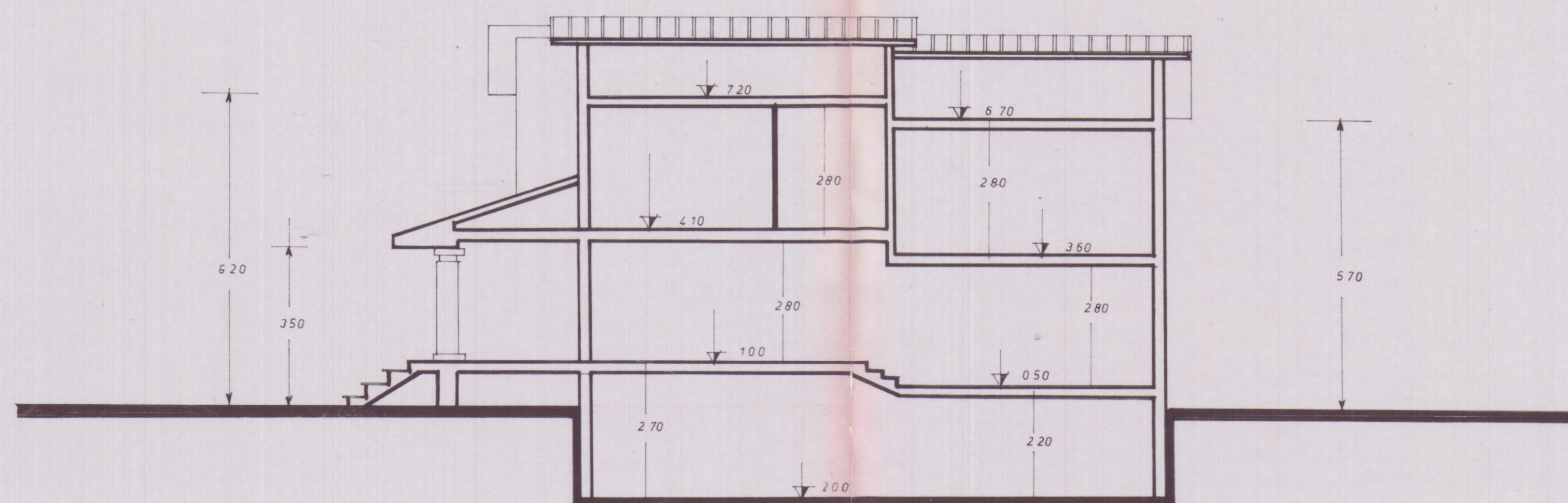
SEZIONE LONGITUDINALE
