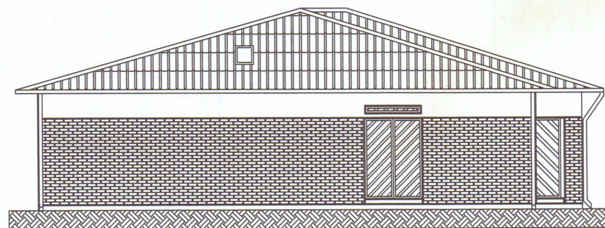
Prospetto SUD-EST
