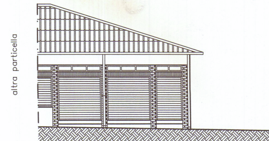
Prospetto SUD-OVEST
