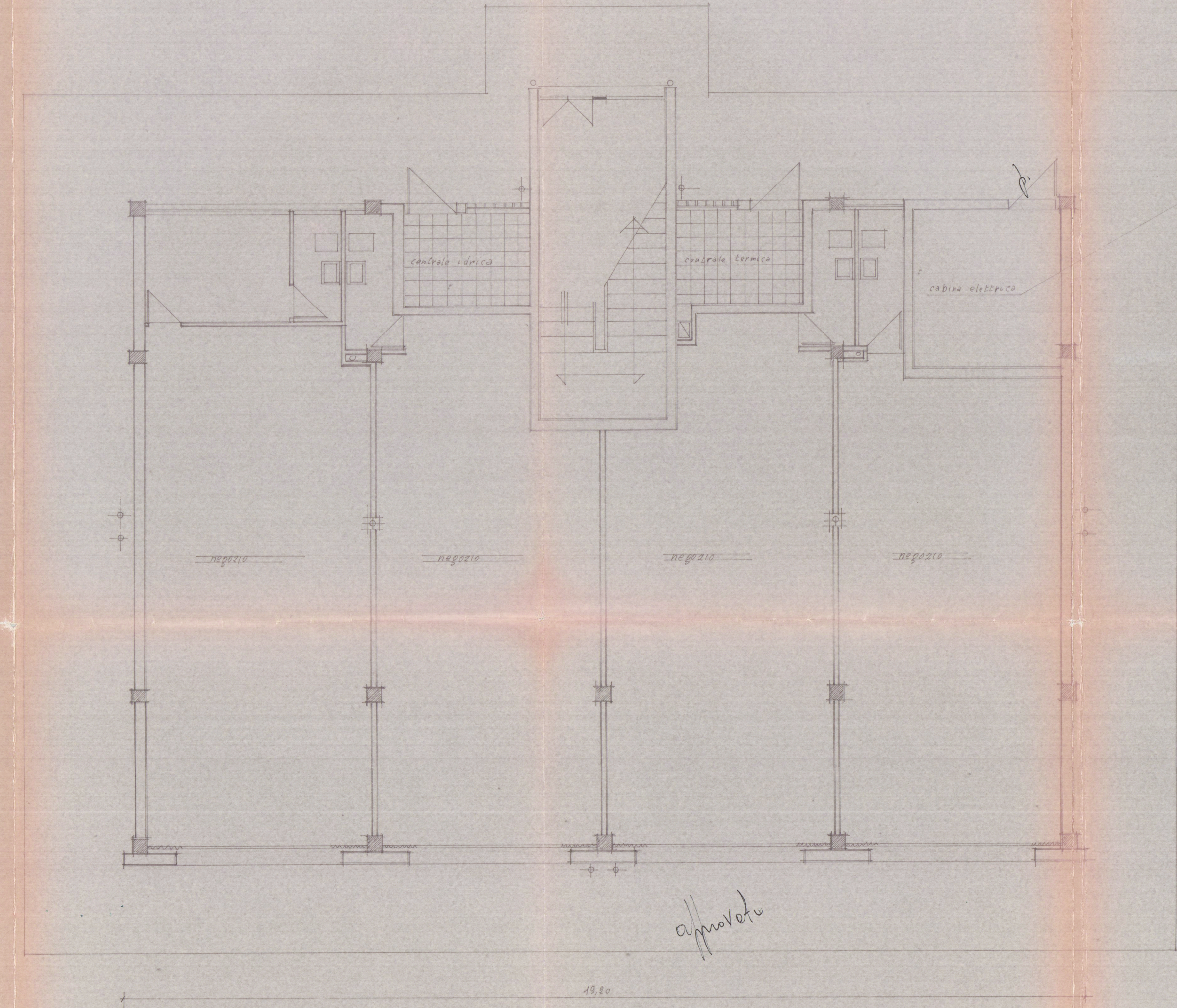
piano terra della variante approvata il 7 agosto 1960 N° 61 protocollo 20235
