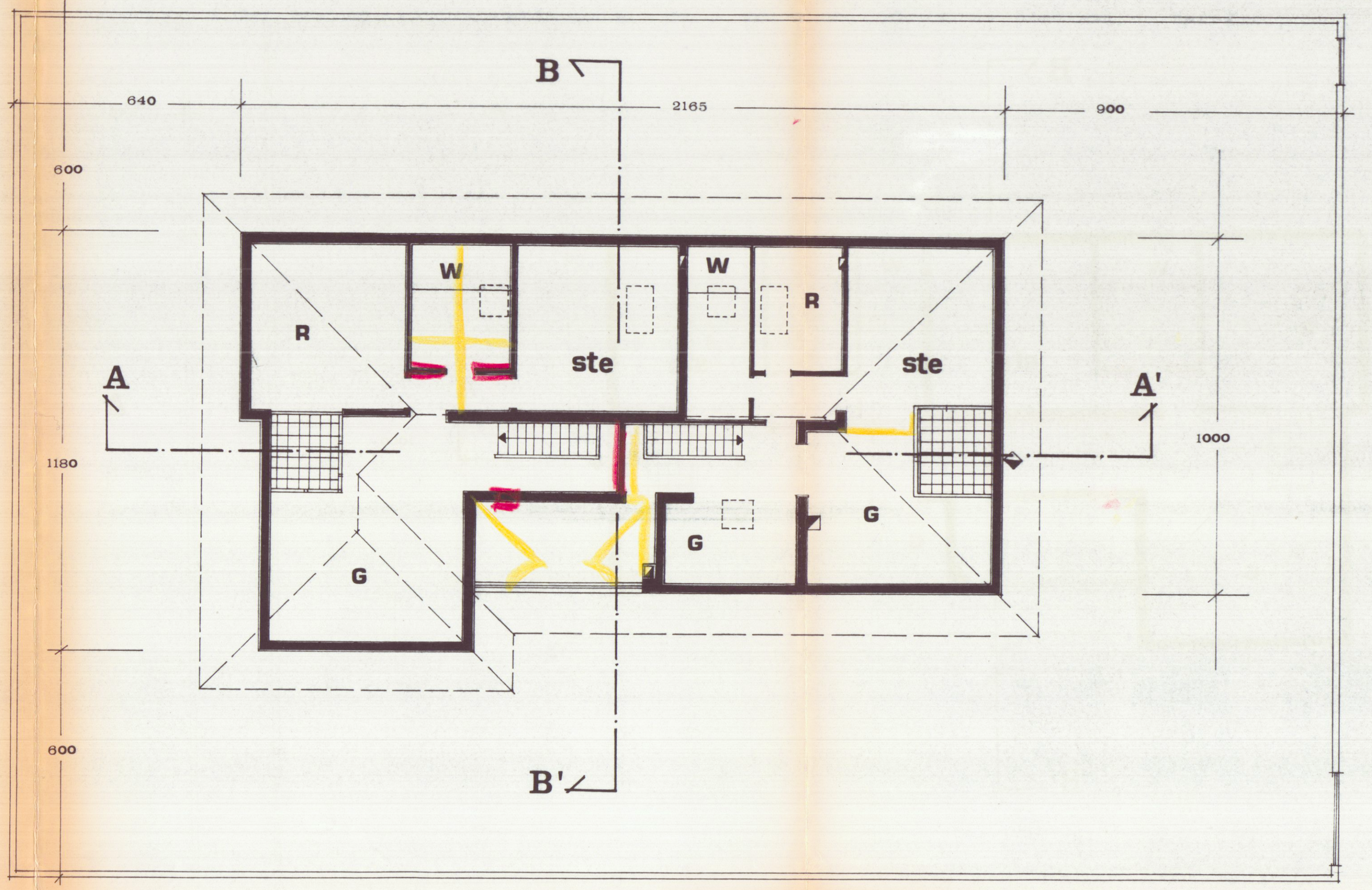
pianta scantinato pianta soffitta
